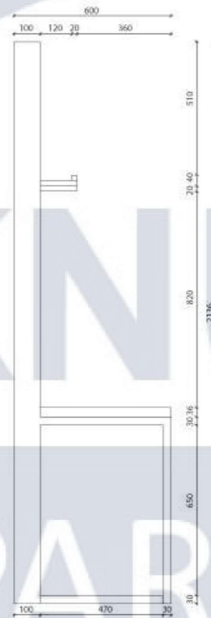
ВИД ЗБОКУ М1:20
