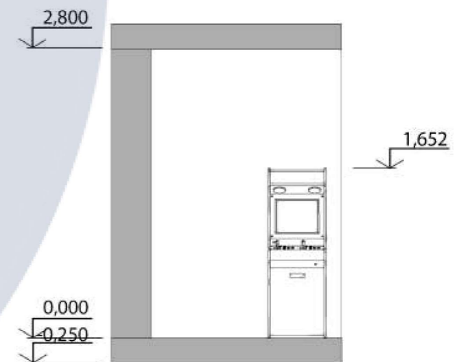
РОЗГОРТКА 13-14
