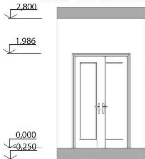
РОЗГОРТКА 14-15
