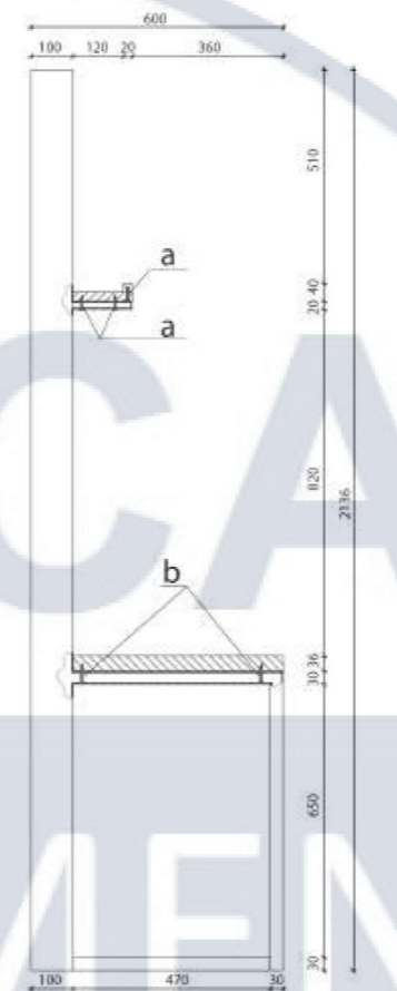
РОЗРІЗ ЗБОКУ М1:20
