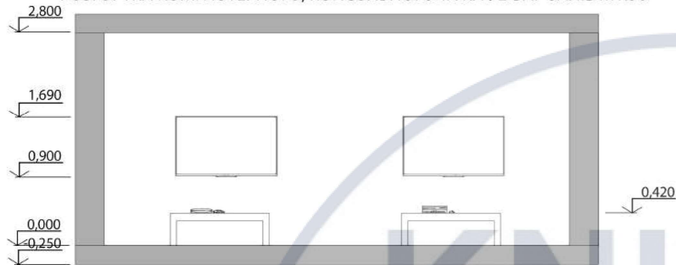
РОЗГОРТКА 8-9
