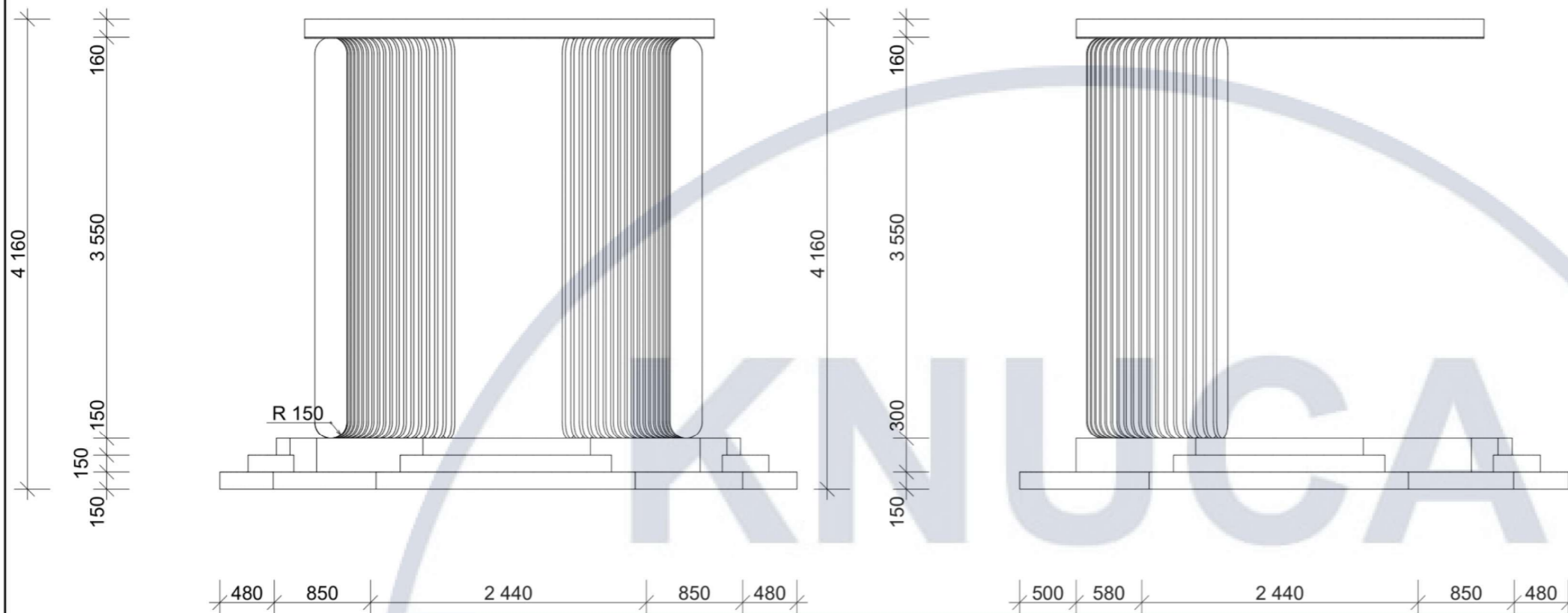
ВИД СПЕРЕДУ М 1:50
