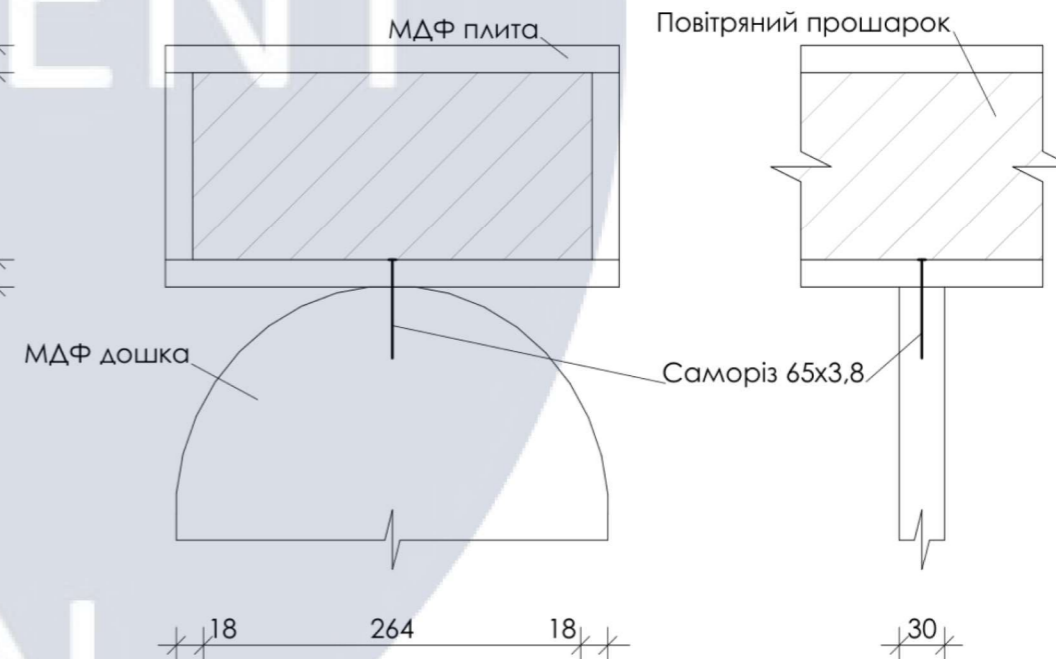
ВУЗОЛ Г М 1:5
