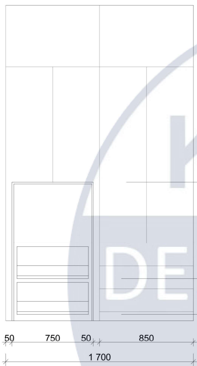
Вид спереду М 1:20
