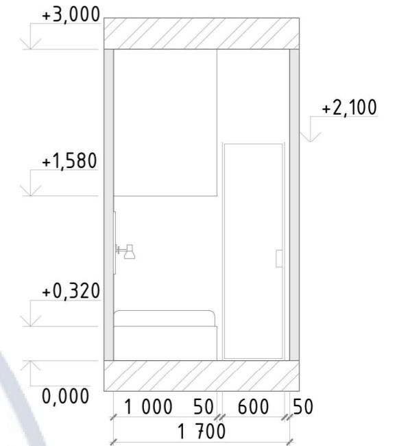
Розгортка 2-3, М 1:50
