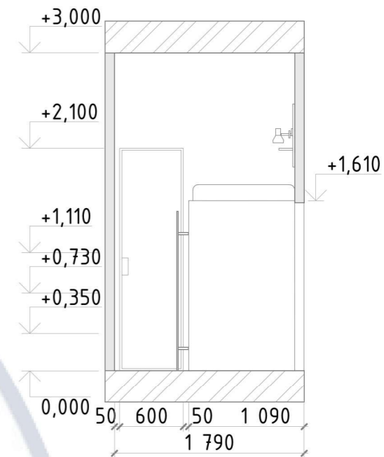
Розгортка 2-3, М 1:50
