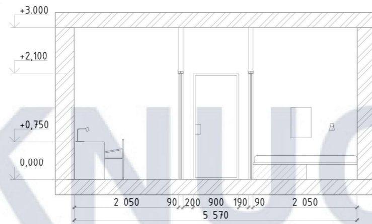
Розгортка 1-2, М 1:75
