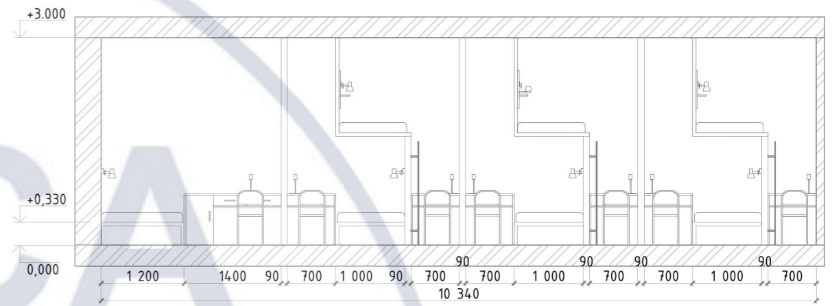
Розгортка 2-3, М 1:75
