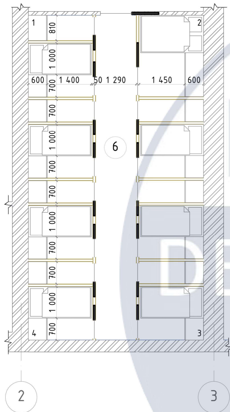
План розташування меблів та обладнання кімнати з капсулами, М 1:75
