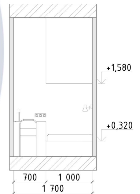
Розгортка 4-1, М 1:50
