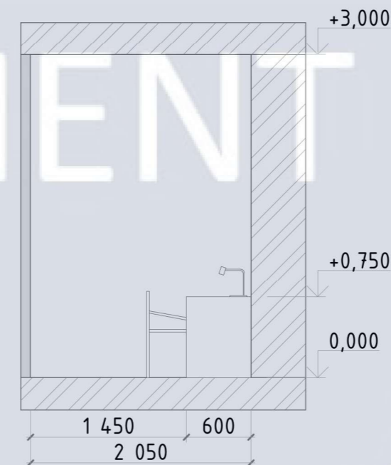
Розгортка 3-4, М 1:50
