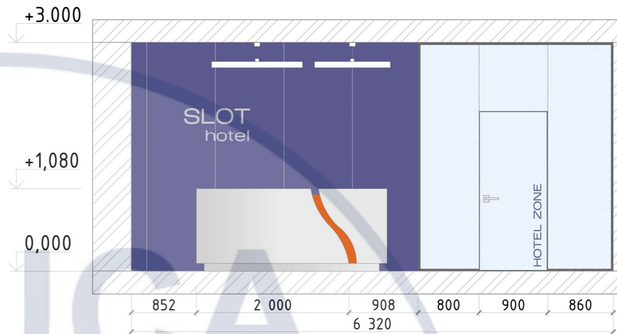
Розгортка 2-3, М 1:50
