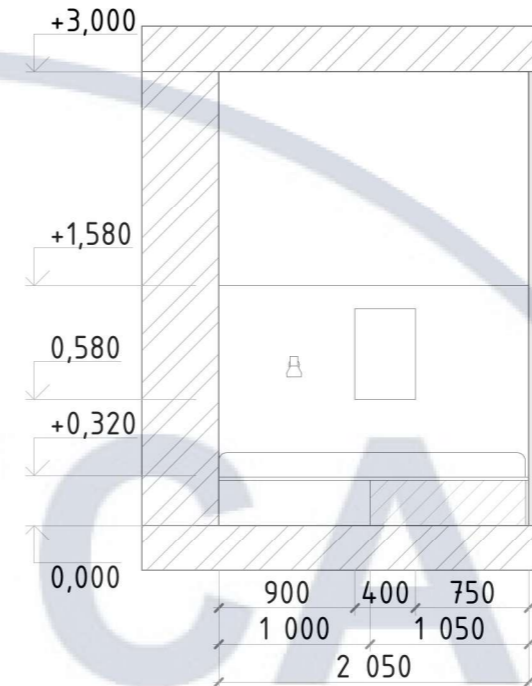
Розгортка 1-2, М 1:50
