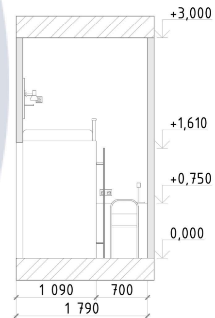
Розгортка 4-1, М 1:50
