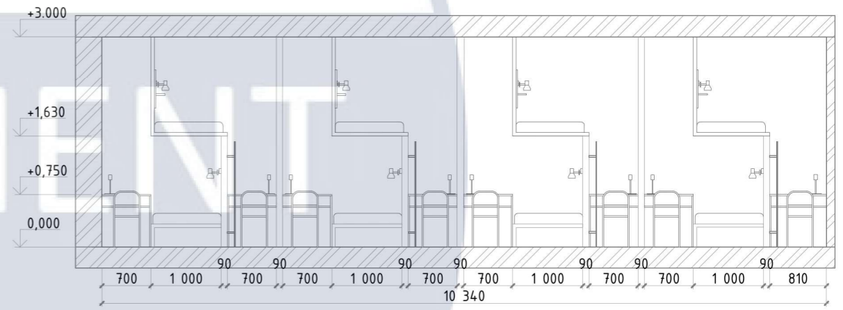
Розгортка 4-1, М 1:75
