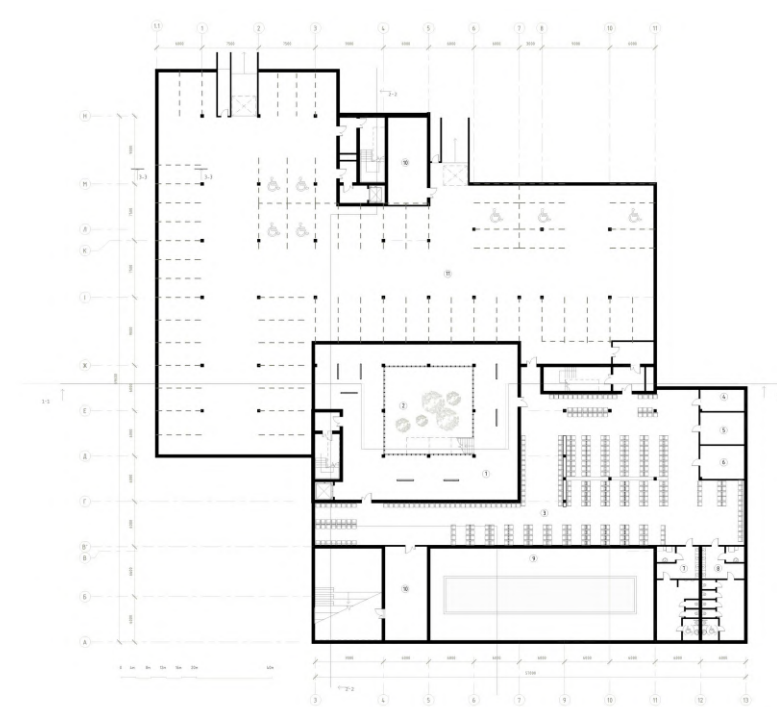
ПЛАН НА ВІДМІТЦІ -3.300
