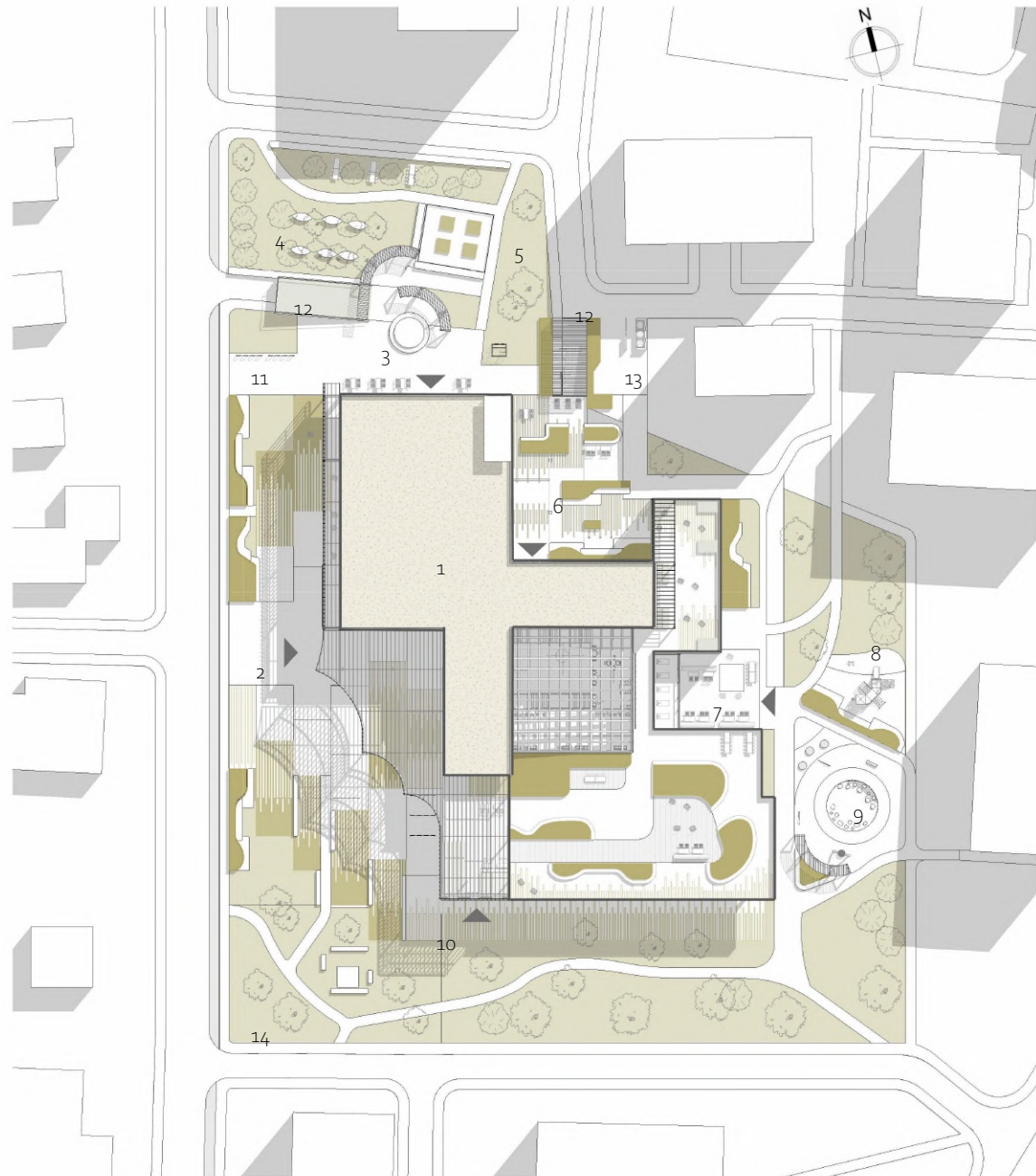
ГЕНЕРАЛЬНИЙ ПЛАН
