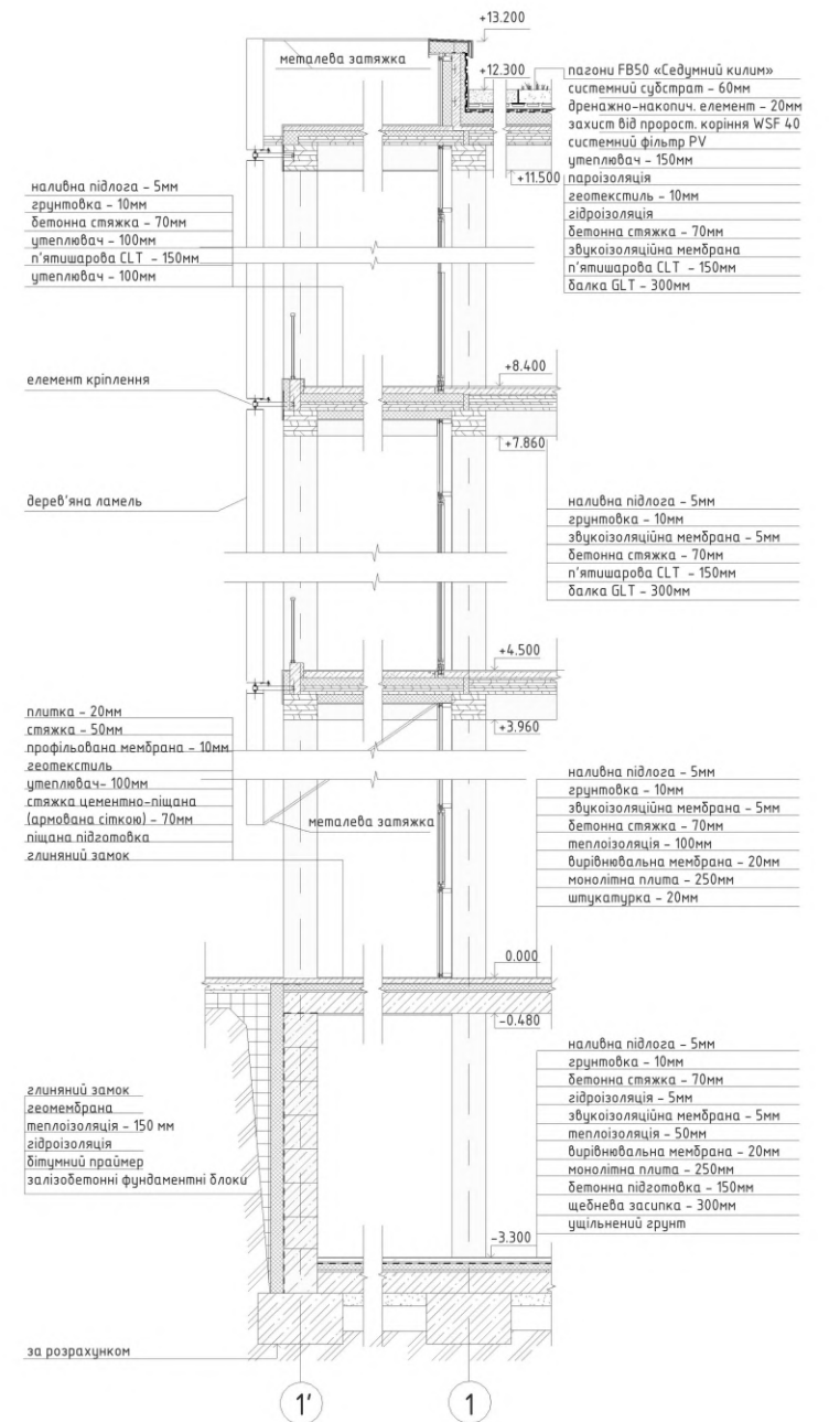
РОЗРІЗ 3-3
