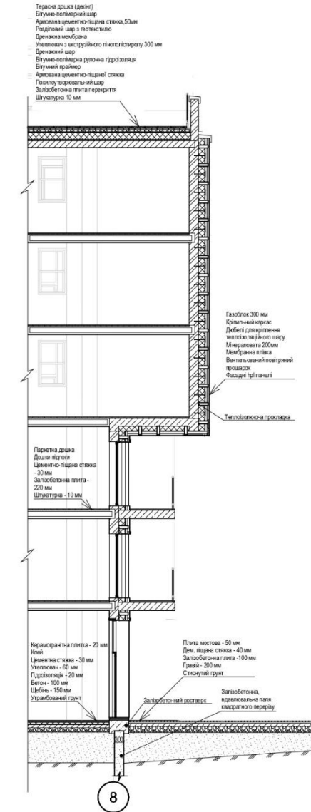
Розріз по стіні
