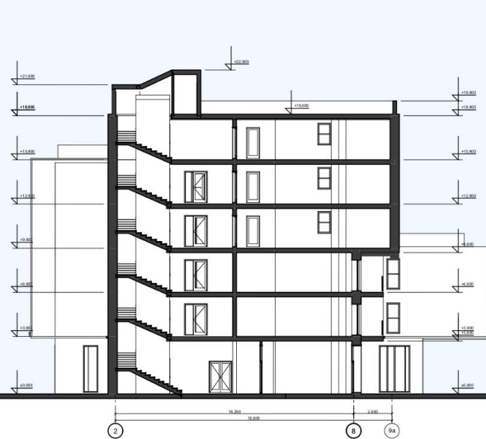
Розріз 1-1'
