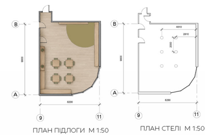
ПЛАН ПІДЛОГИ М 1:50
