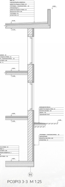
РОЗРІЗ 3-3 М 1:25
