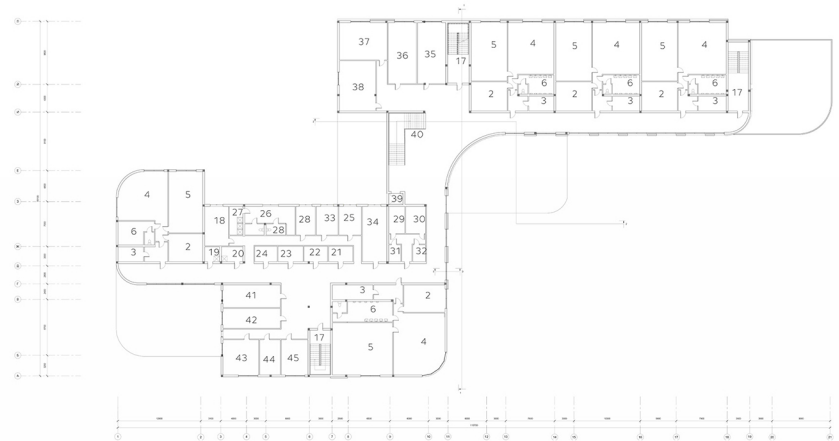
ПЛАН НА ВІДМІТЦІ +3.500 М 1:100
