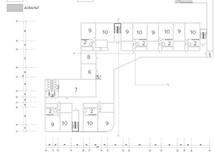
ПЛАН НА ВІДМІТЦІ -4.500 М 1:200
