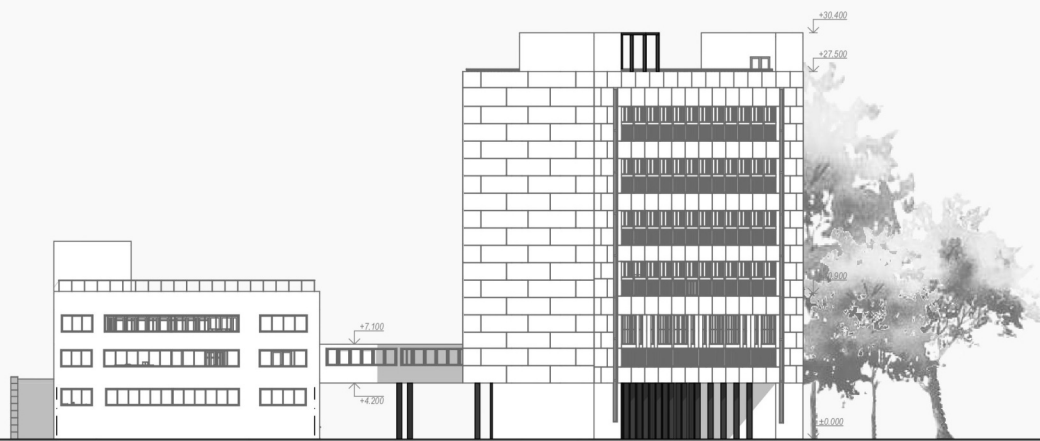
ФАСАД В ОСЯХ А-Г М 1:400
