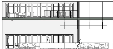
РОЗГОРТКА М 1:200
