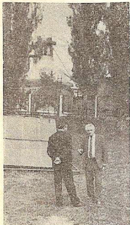
Радгосп «Росія». Фрагмент блоку геїстоколекторів. На задньому плані — біогазова установка.
