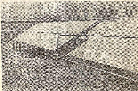
Черкаська область. Радгосп «Росія». Геїстоустановка з колекторами Братського заводу.
