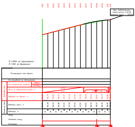
Поздовжній профіль районної магістрали 2 по вул. Срібняківська
