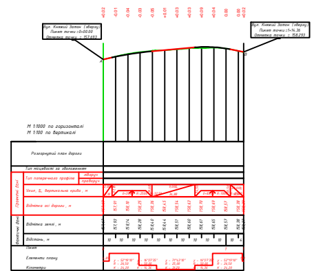
Поздовжній профіль районної магістрали 1-3 ( по вул. Кижий Заман
