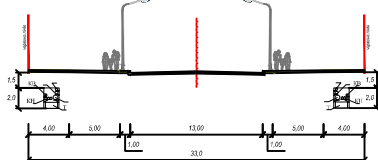
Проектний поперечний профіль магістралі районного значення 2 по вул. Сербійській М 1:200
