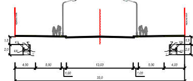
Проектний поперечний профіль магістралі районного значення 1-3 по вул. Ювілейній Замості М 1:200
