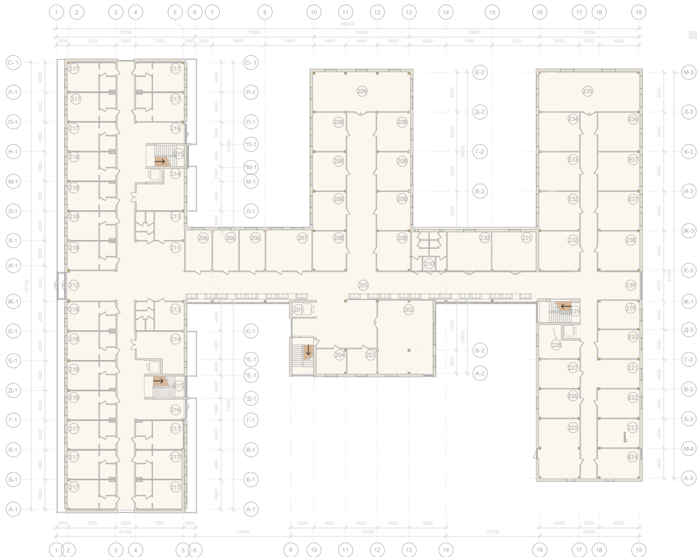
План на відмітці +3,600
