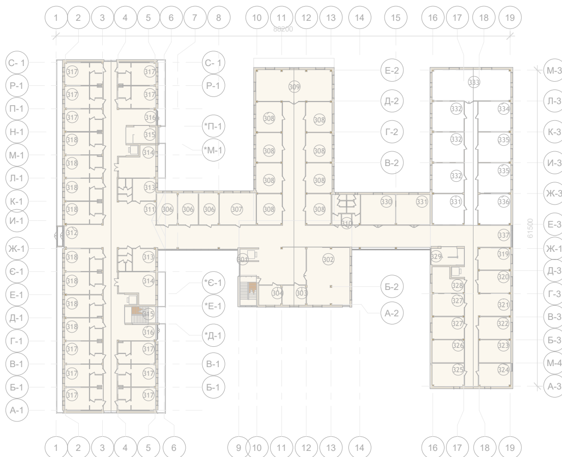
План на відмітці +7,200
