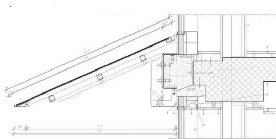
Вузол кріплення в розрізі сонцезахисного козирька М 1:20
