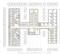
План на відмітці +7,200
