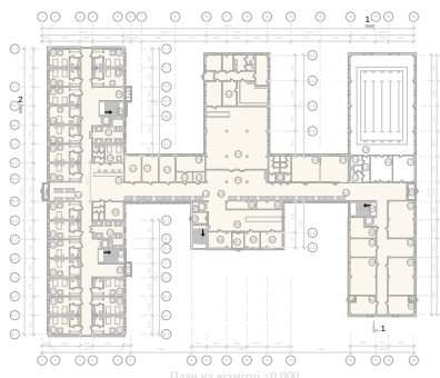
План на відмітці +0,000
