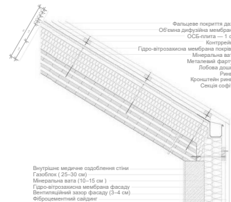
Вузол 2 М 1:20
