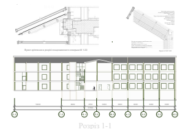
Розріз 1-1
