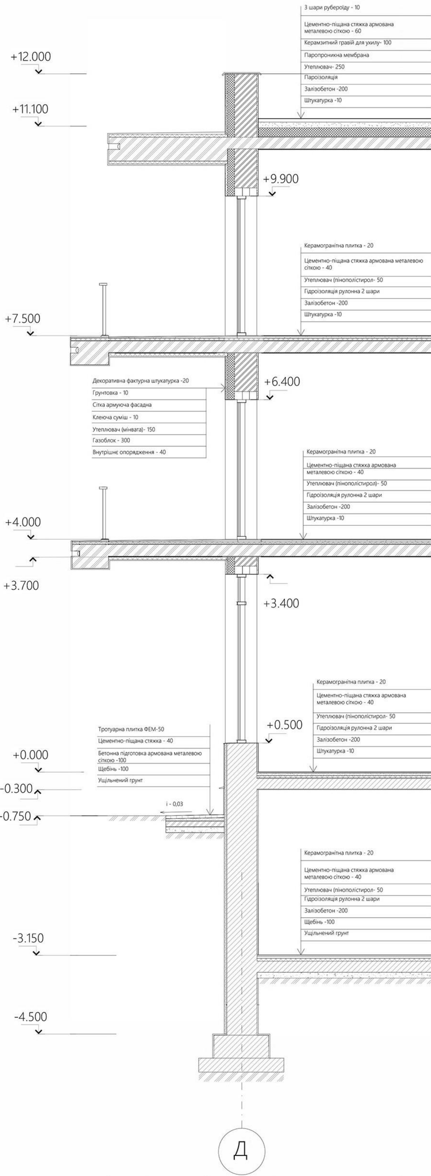
РОЗРІЗ 3-3 М 1:20
