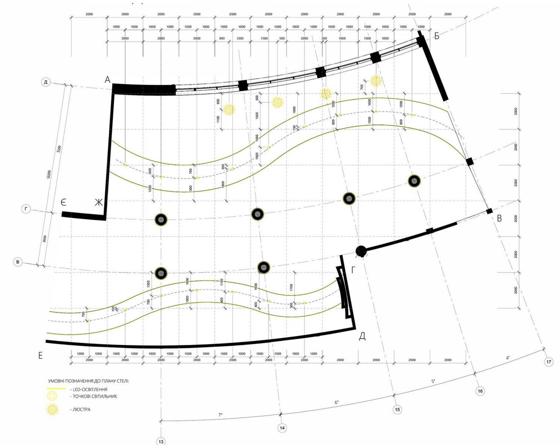
ПЛАН СТЕЛІ М 1:50
