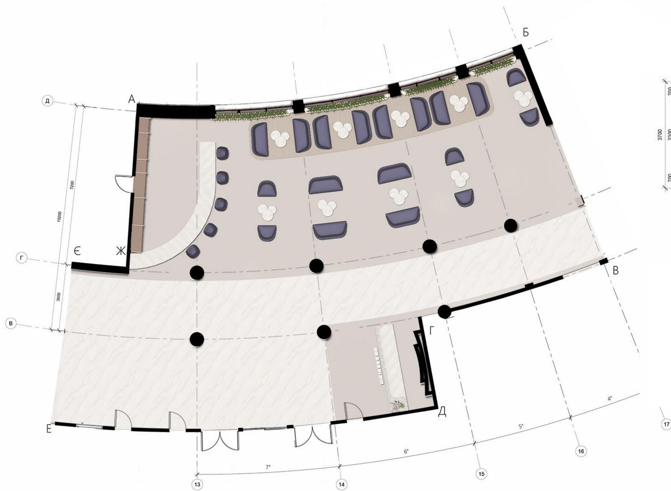
ПЛАН ПІДЛОГИ М 1:50
