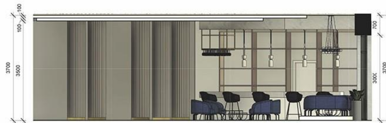
РОЗГОРТКА Е-А М 1:50
