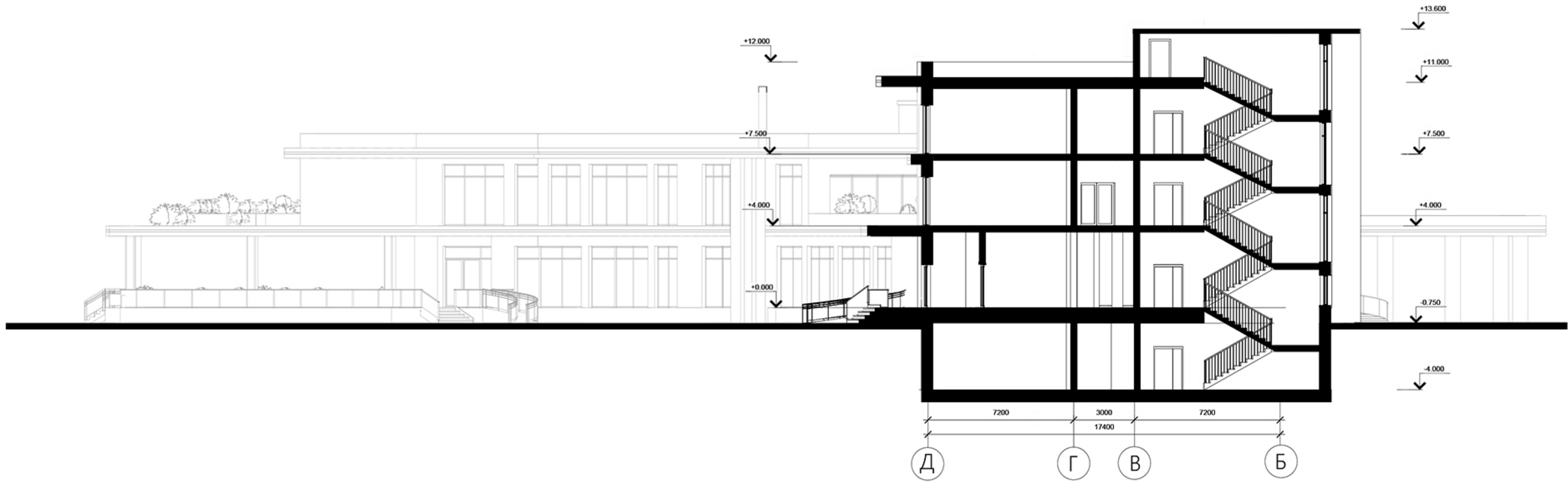
РОЗРІЗ 1-1 М 1:100
