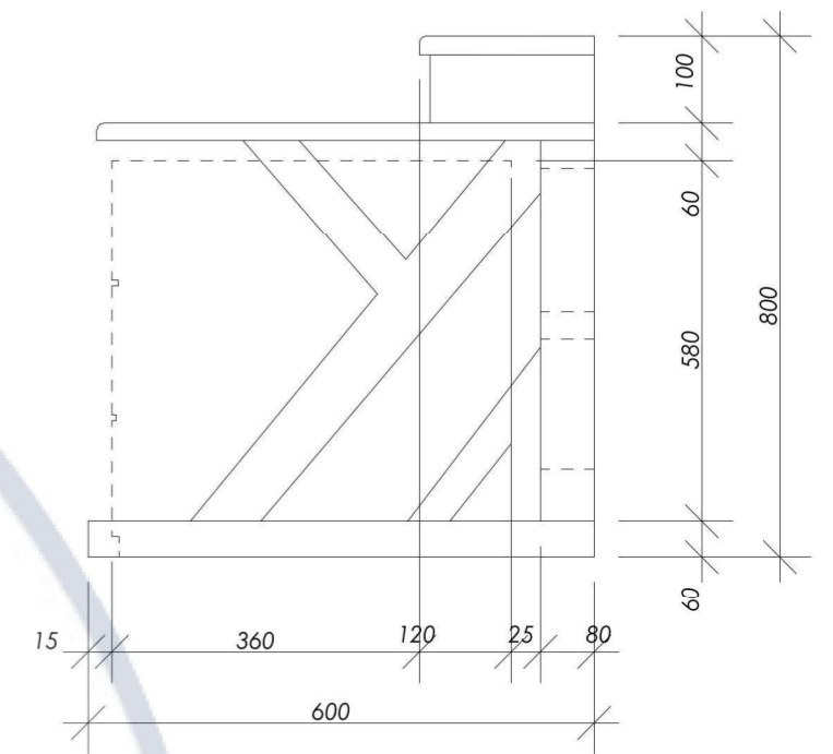
Вид збоку М 1:10
