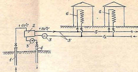
Мал. 1. Схема системи теплопостачання з використанням термальних вод. 1 — свердловина термальних вод; 2 — тепловий насос; 3 — циркуляційний насос; 4 — свердловина для закачування води; 5 — зовнішня теплова мережа; 6 — система опалення будинка.
