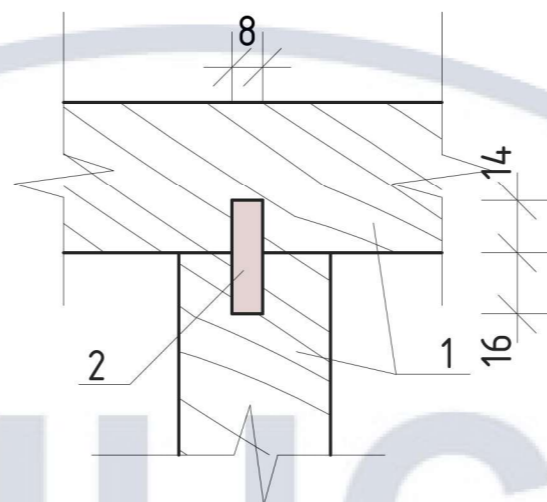
Вузол 1
