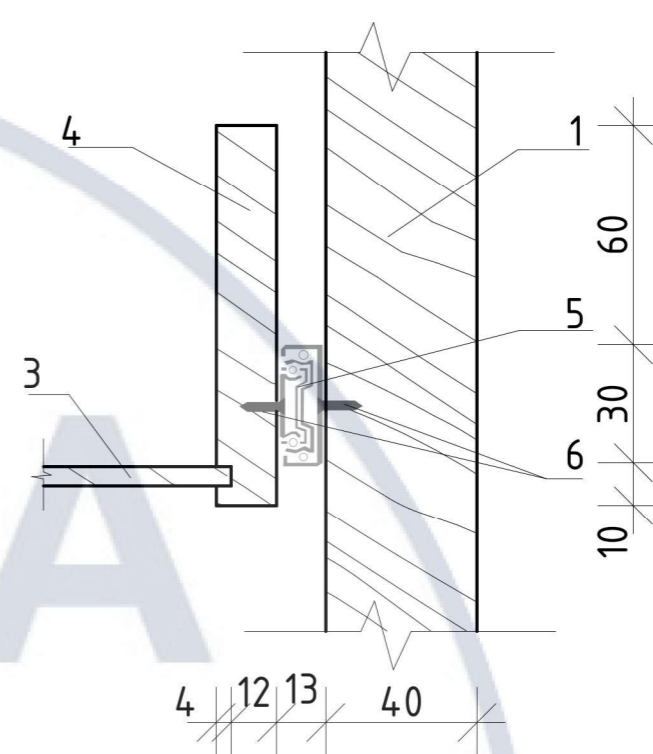
Вузол 2
