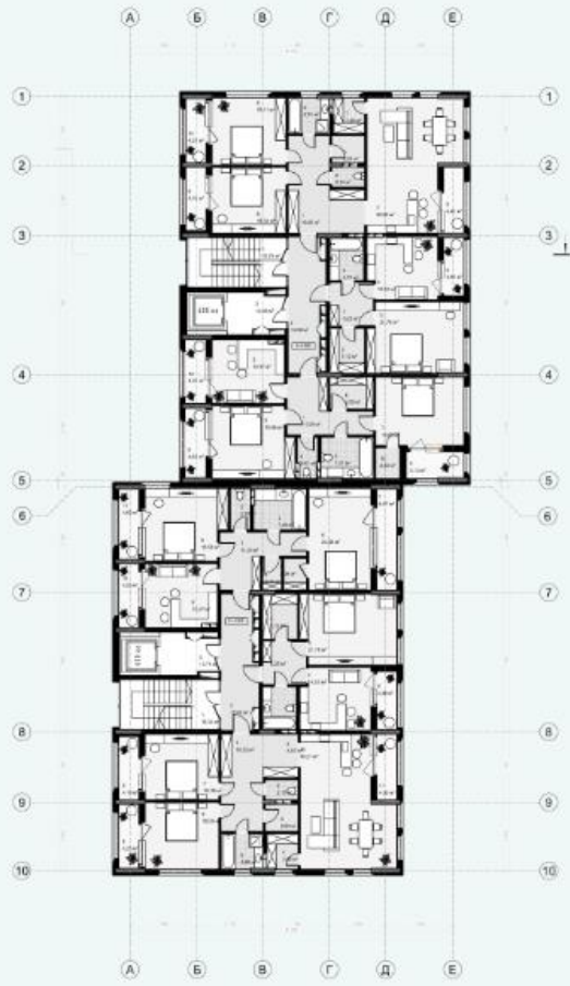
План 2-го поверху будинку №2 на відмітці 3.500 М1:100
