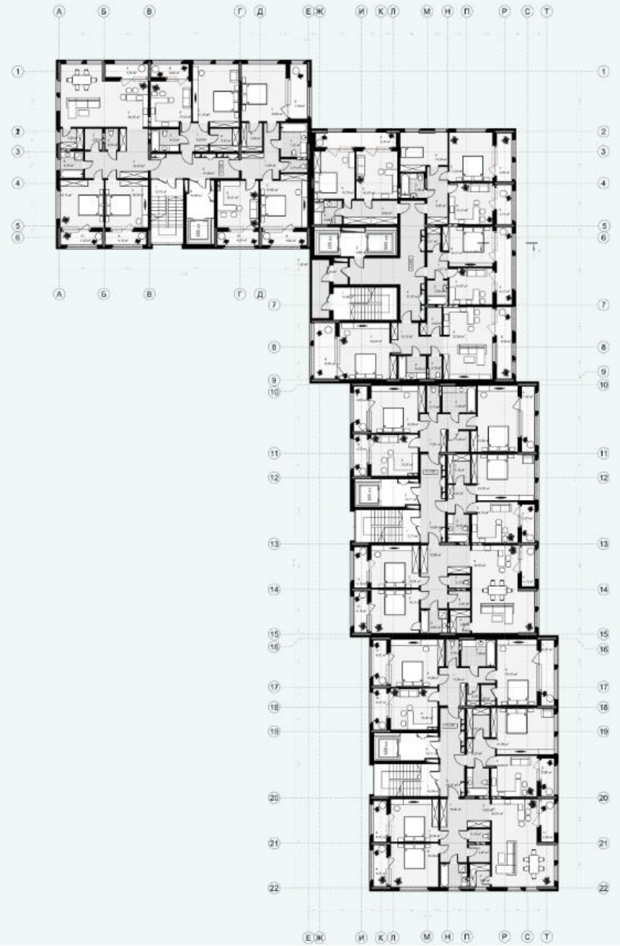
План 2-го поверху будинку №1 на відмітці 3.500 М1:100
