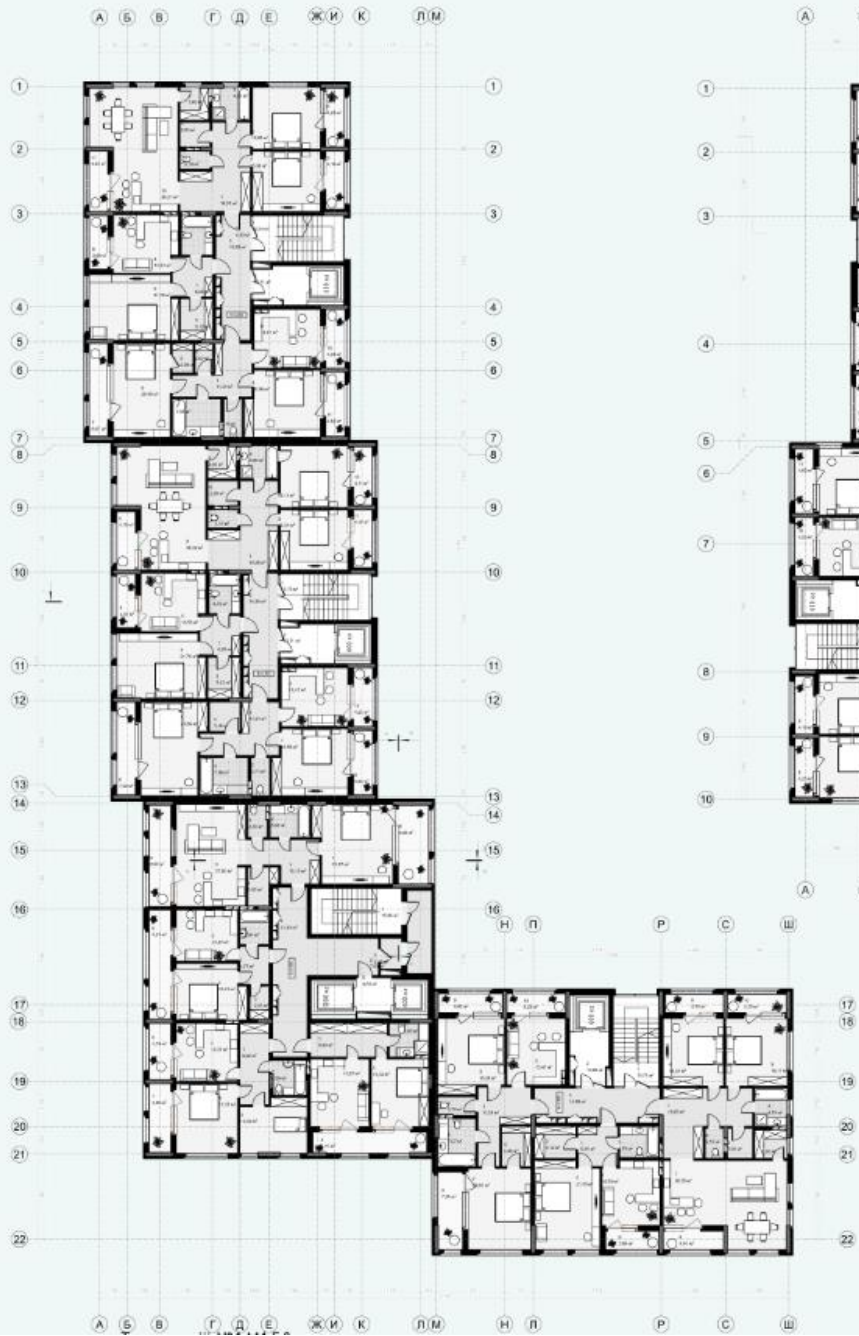
План 2-го поверху будинку №3 на відмітці 3.500 М1:100
