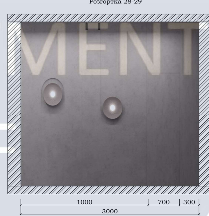
Розгортка 31-31
