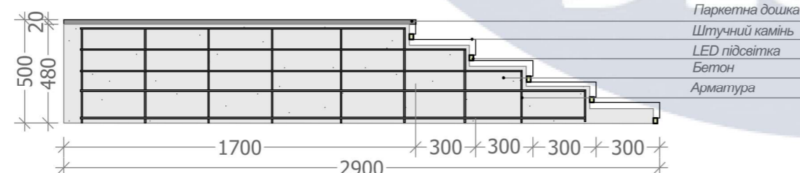
Конструкція платформи М1:20
