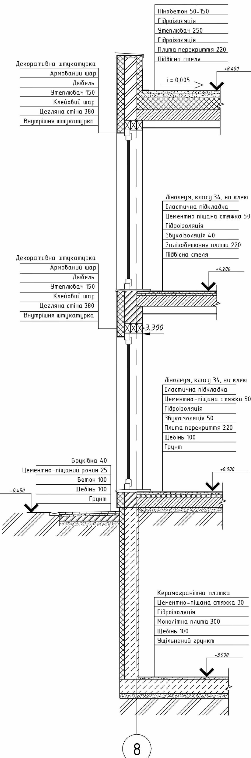
Розріз 3 – 3 М 1:50
