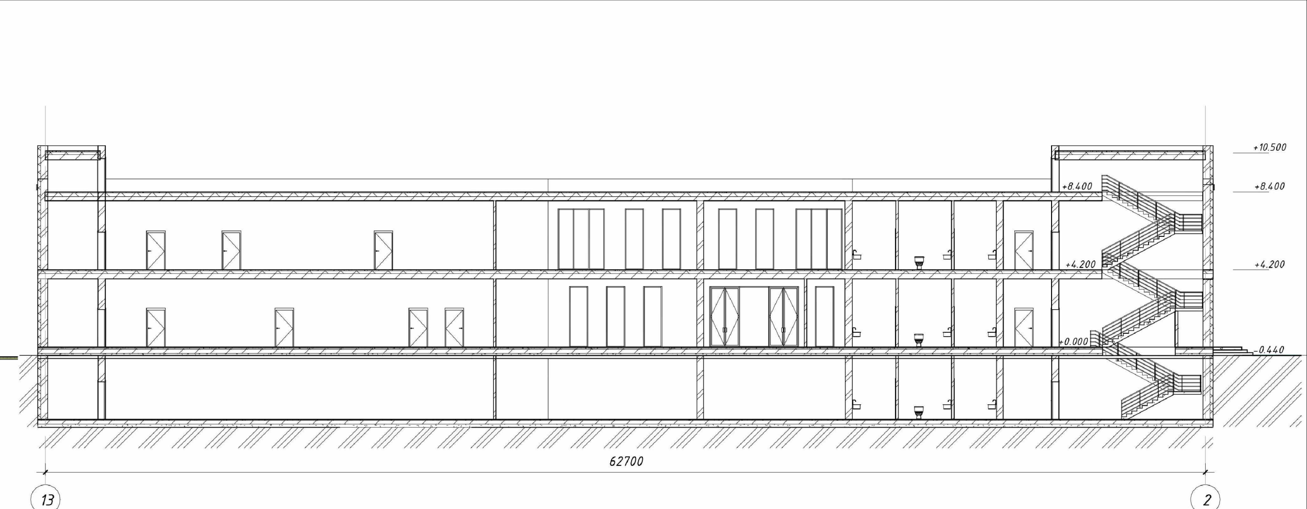
Розріз 1 – 1 М 1:200
