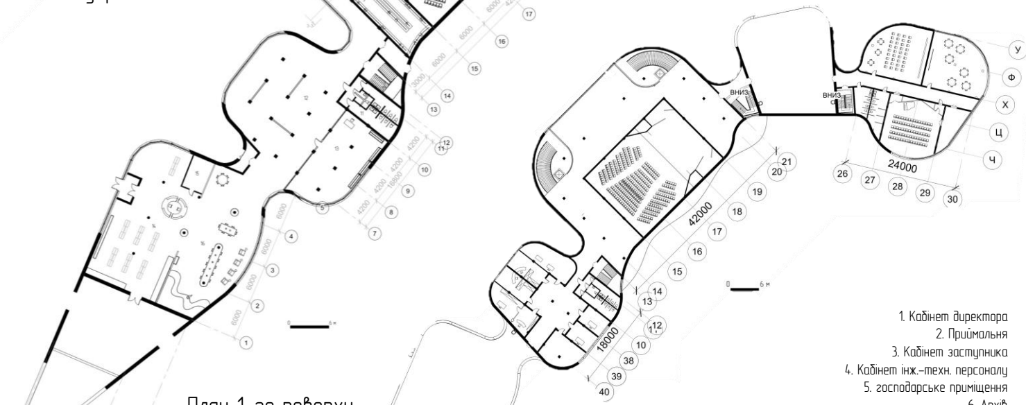
План 1-го поверху
