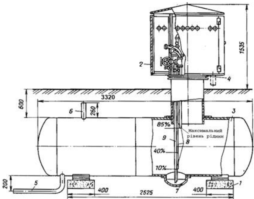
Рис. 3.3 Установка резервуару ємкістю 2,5 м 3 :
