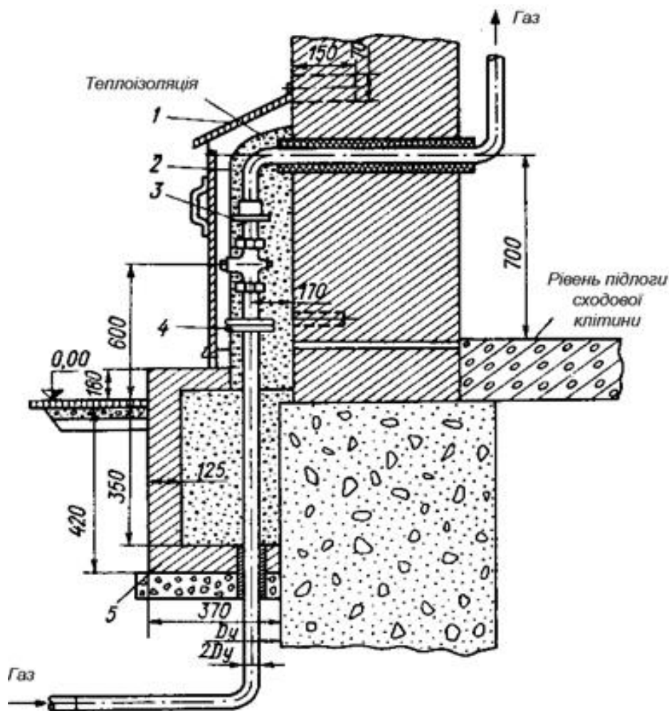
Рис. 5.1. Утеплений ввід газопроводу СВГ [15]:
