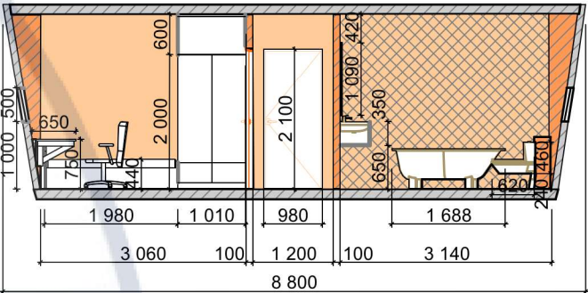
Розгортка Б-В М 1:100
