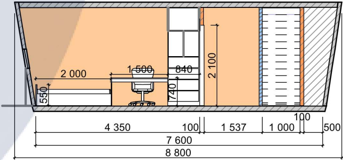
Розгортка Г-А М 1:100
