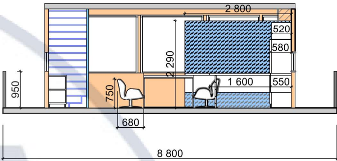
Розгортка 2-3 М 1:100
