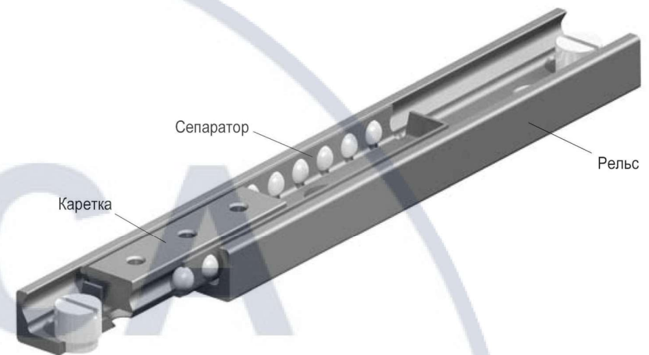
Вузол 1
