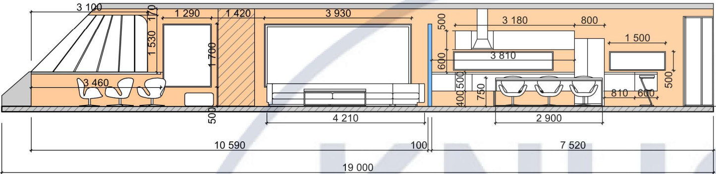
Розгортка 1-2 М 1:100
