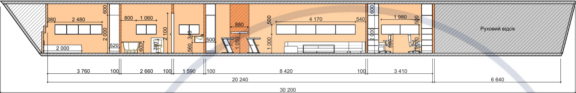
Розгортка А-Б М 1:100
