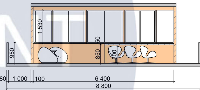
Розгортка 4-1 М 1:100
