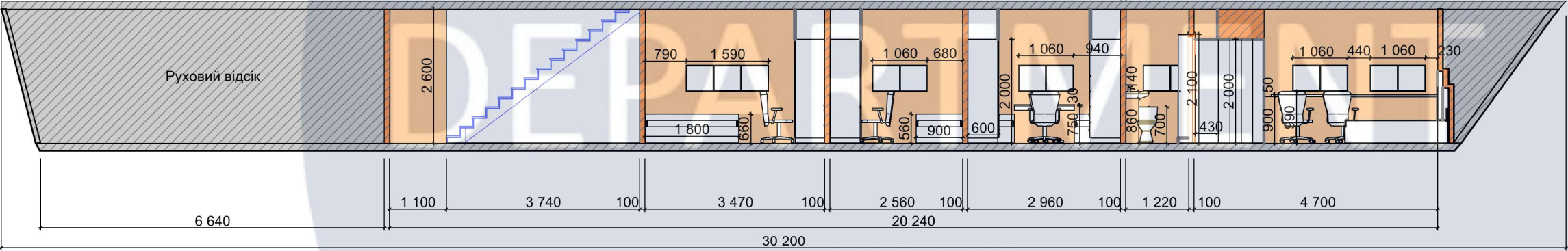
Розгортка В-Г М 1:100
