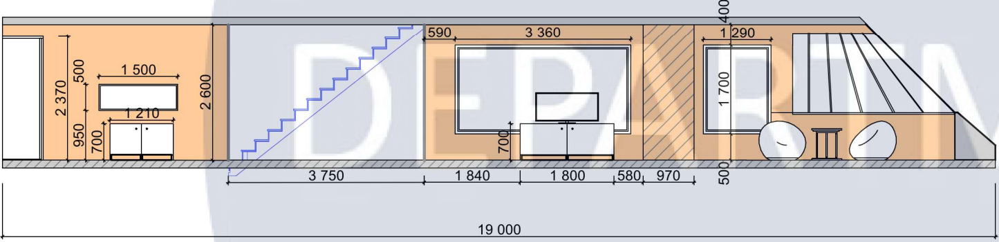
Розгортка 3-4 М 1:100
