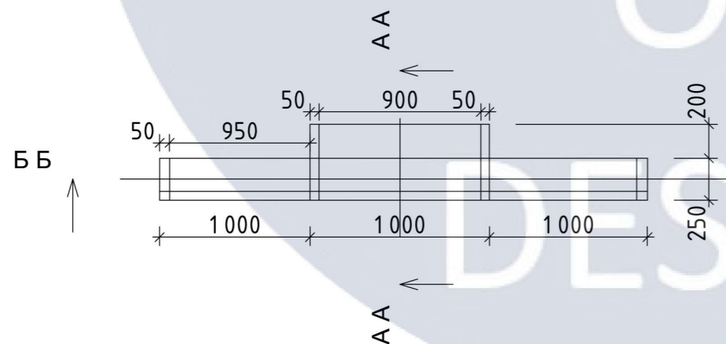
Вид зверху
