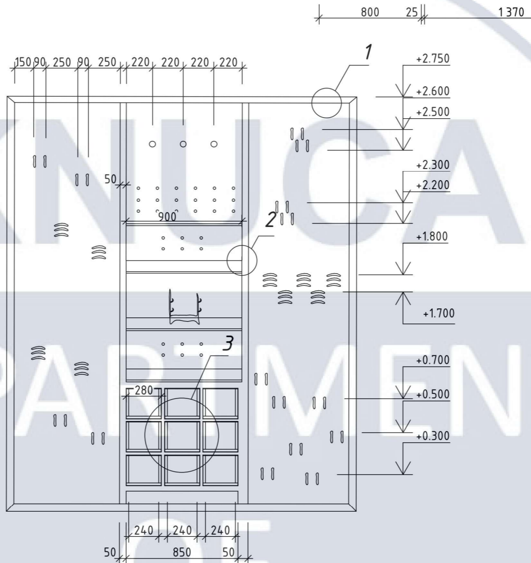
Розріз Б - Б
