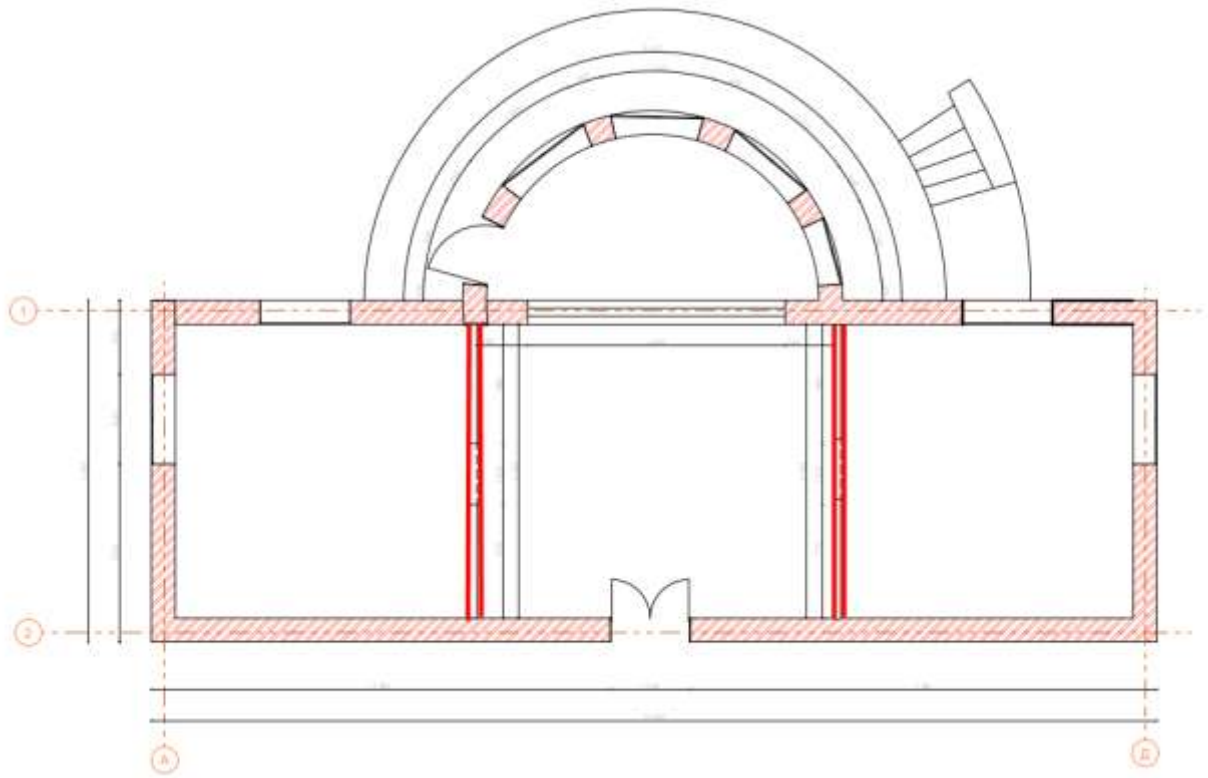
Рис 2.3 План демонтажу
