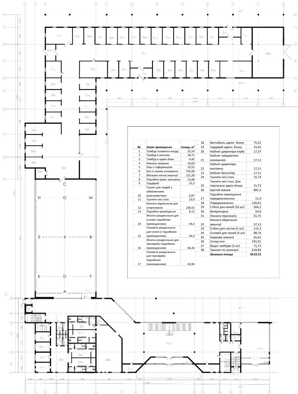
План першого поверху
