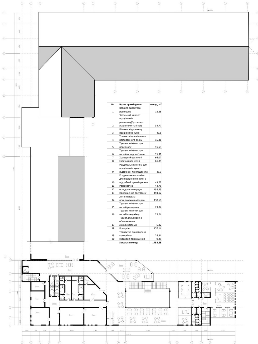
План другого поверху
