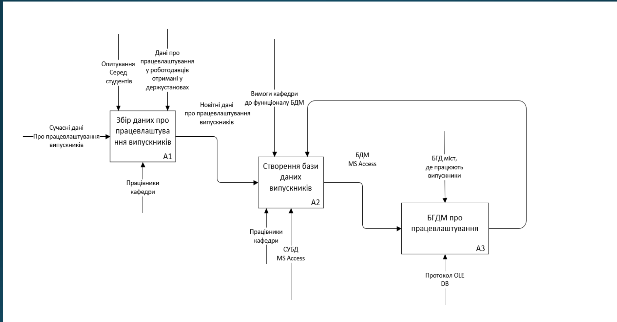
Рис.4. Узагальнена контекстна IDEF0-діаграма технології побудови бази геоданих системи моніторингу працевлаштування випускників кафедри
