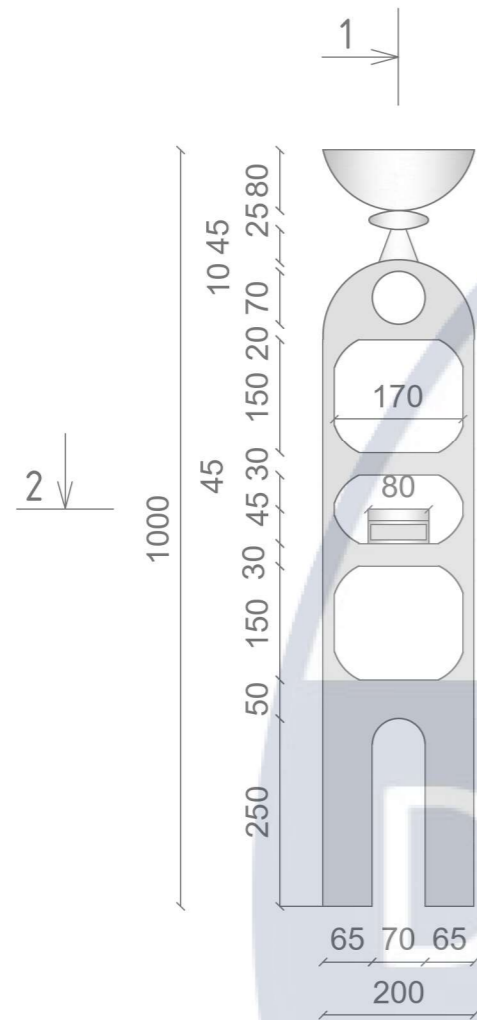
Фронтальна проєкція
