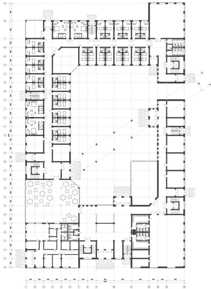
План першого поверху
