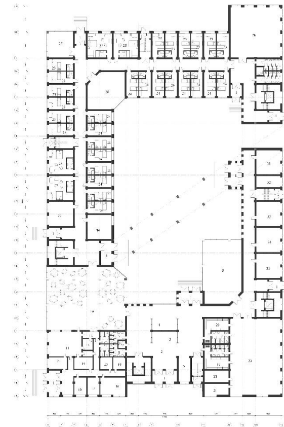
План поверху
