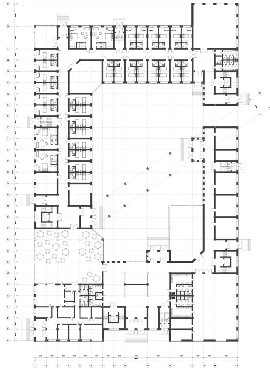
План першого поверху
