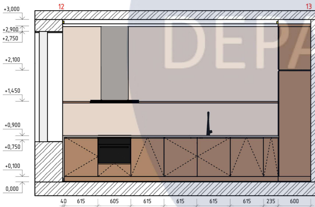
Розгортка 12-13 M1:40
