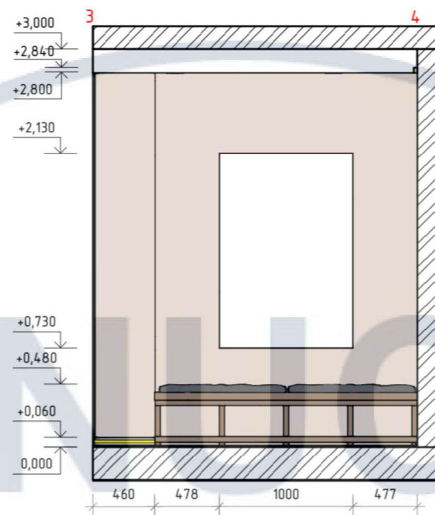
Розгортка 3-4 M1:40
