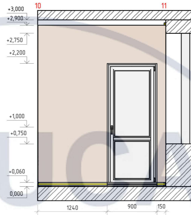
Розгортка 10-11 M1:40
