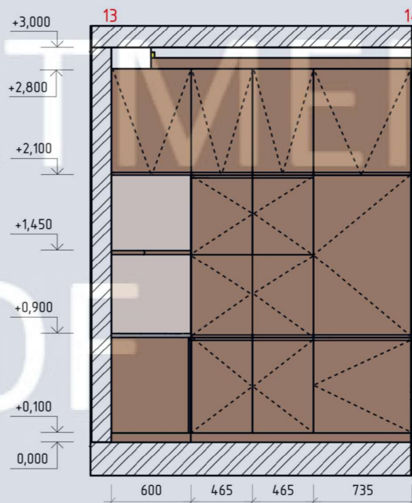
Розгортка 13-14 M1:40
