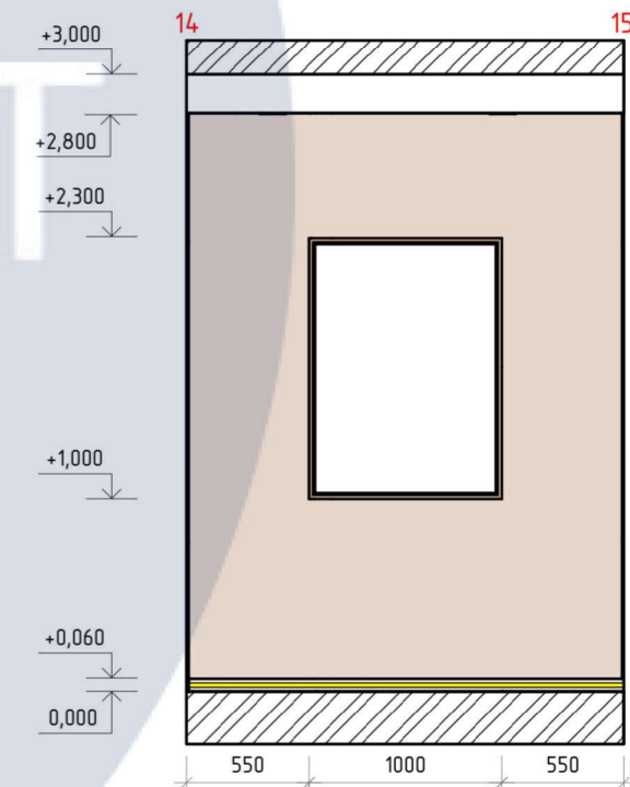
Розгортка 14-15 M1:40
