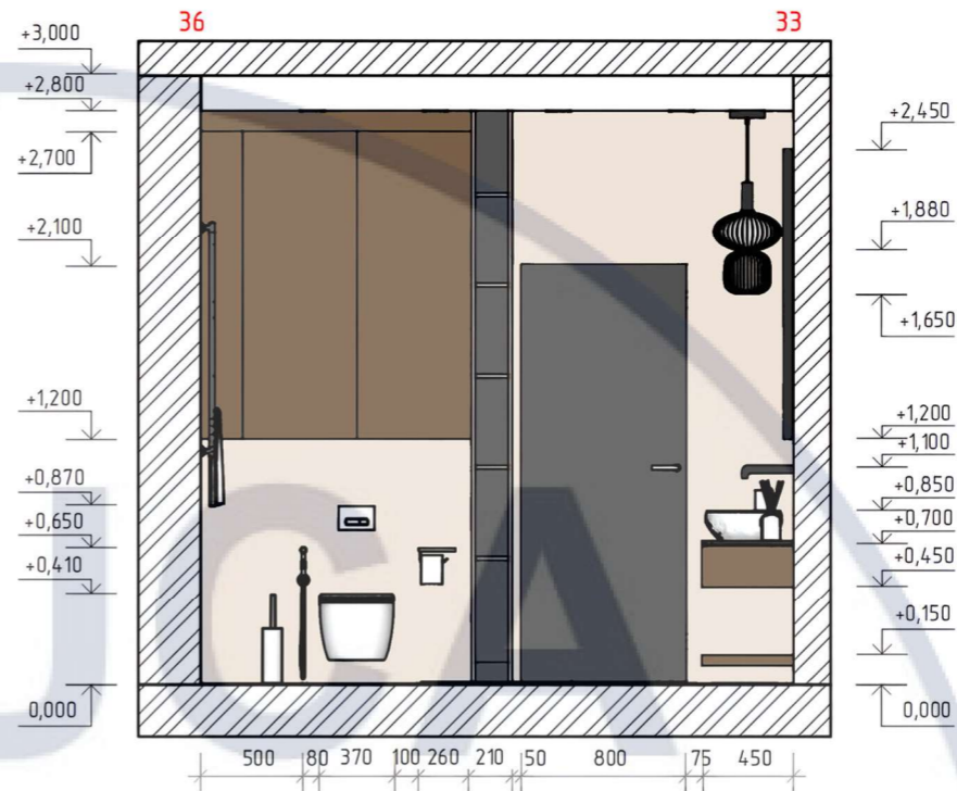
Розгортка 36-33 M1:40
