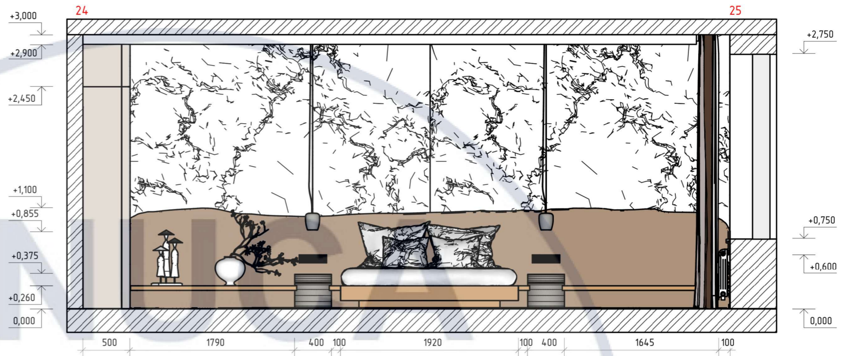
Розгортка 24-25 M1:40
