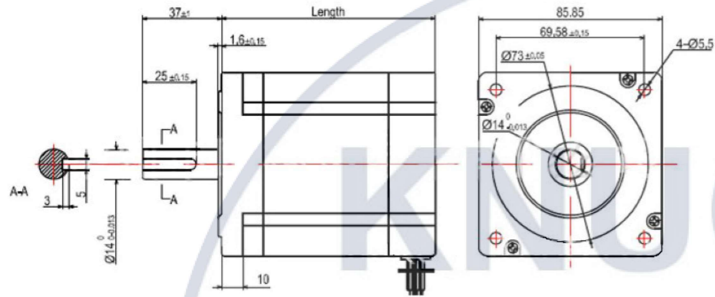
Кроковий двигун Nema 34 (86мм) серії Wantai
