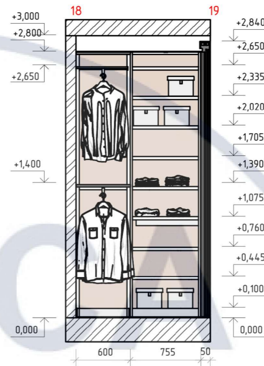
Розгортка 18-19 M1:40
