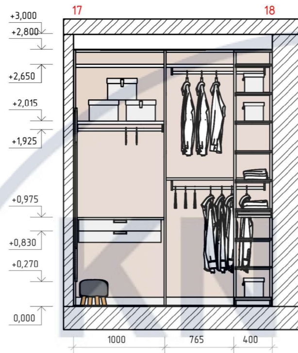
Розгортка 17-18 M1:40
