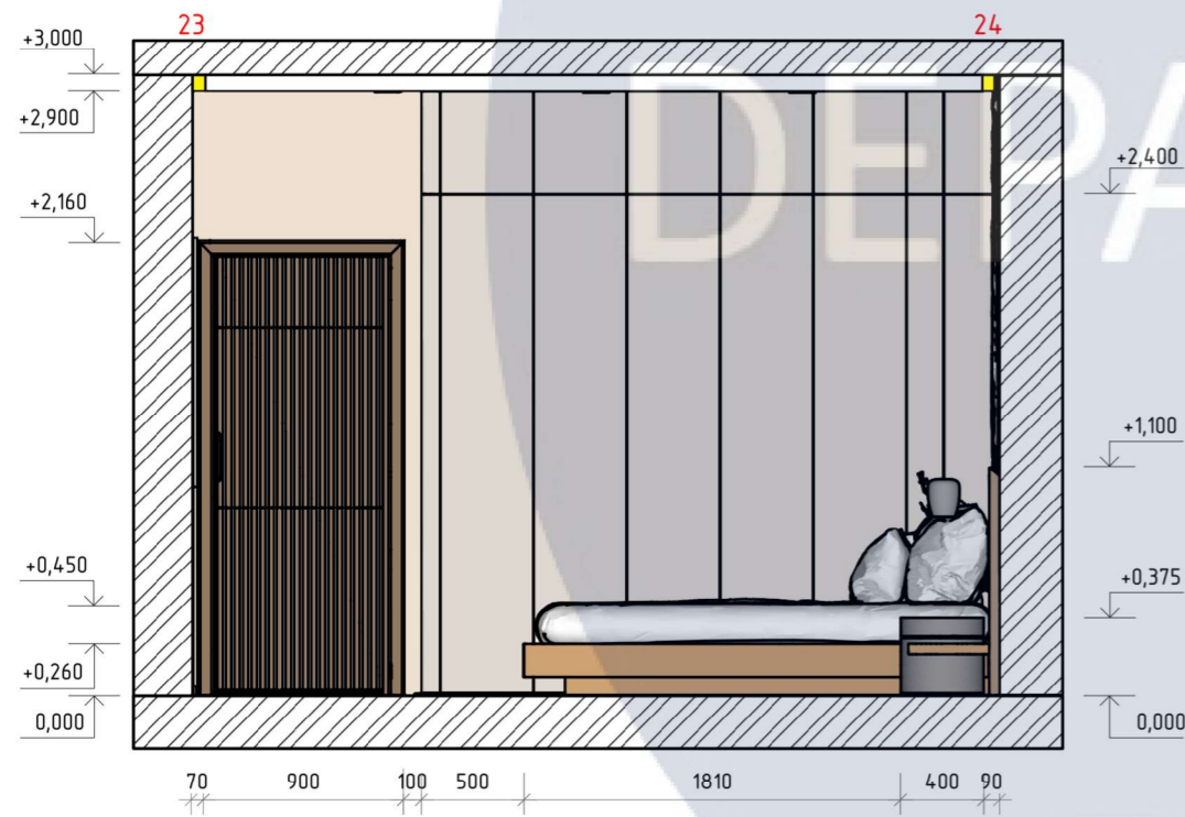
Розгортка 23-24 M1:40
