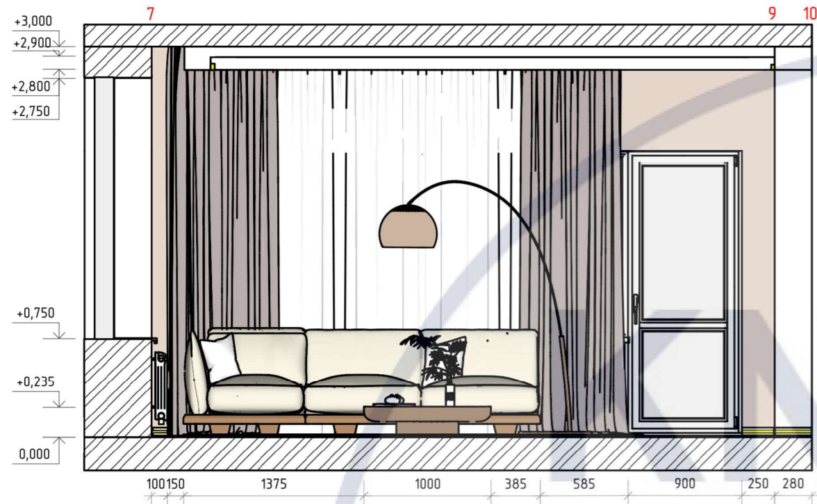
Розгортка 7-10 M1:40
