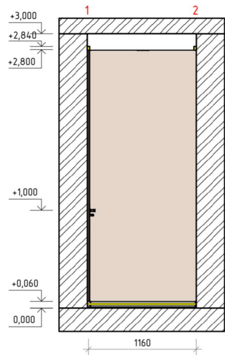
Розгортка 1-2 M1:40
