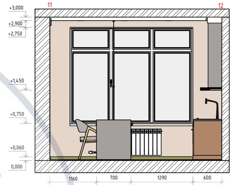
Розгортка 11-12 M1:40
