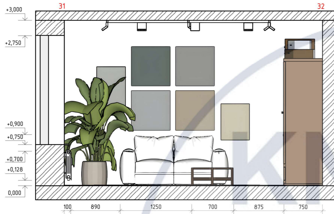
Розгортка 31-32 М1:40
