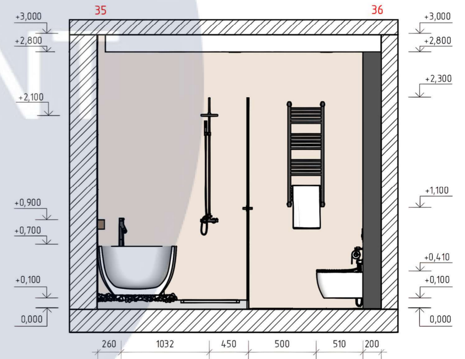
Розгортка 35-36 M1:40
