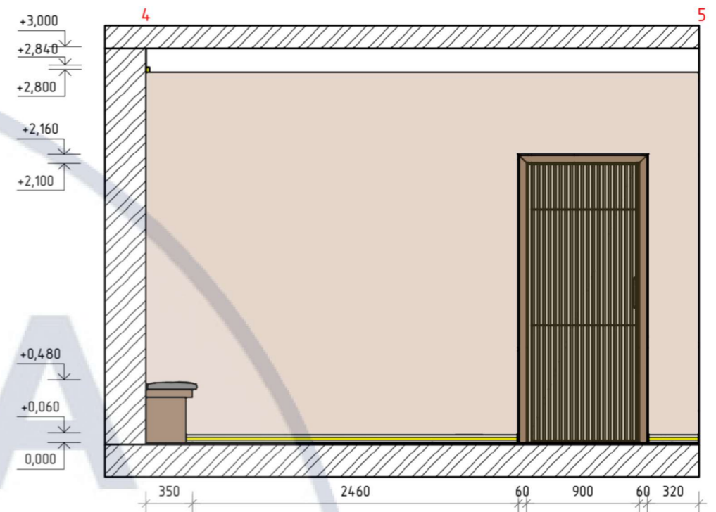
Розгортка 4-5 M1:40
