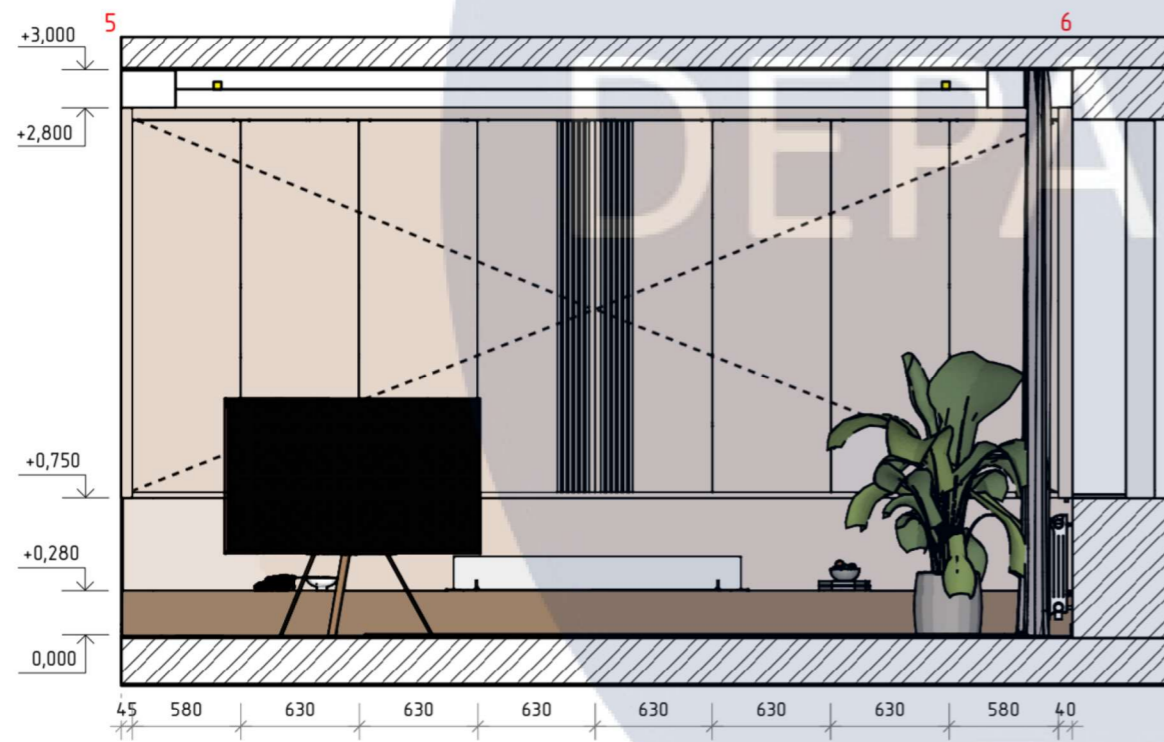
Розгортка 5-6 M1:40
