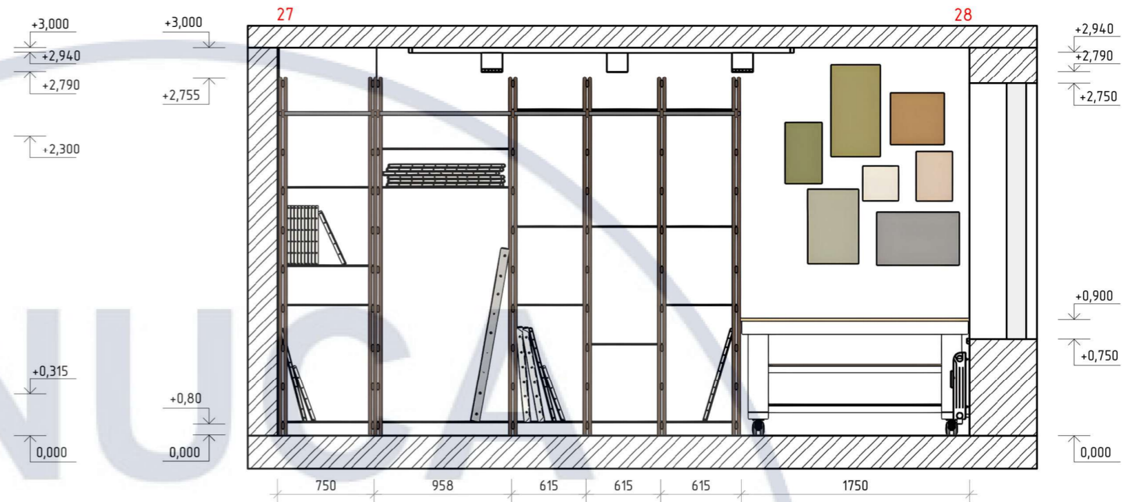
Розгортка 27-28 М1:40
