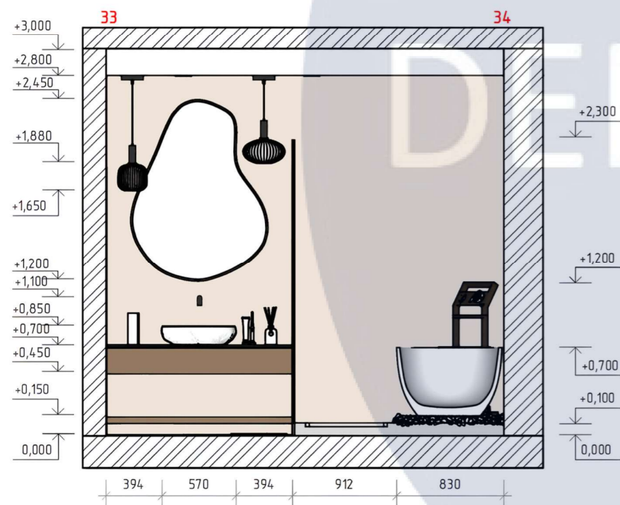
Розгортка 33-34 M1:40
