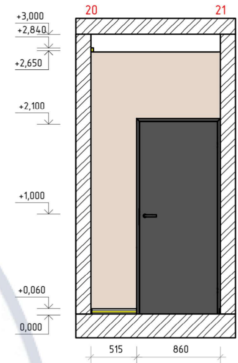
Розгортка 20-21 M1:40
