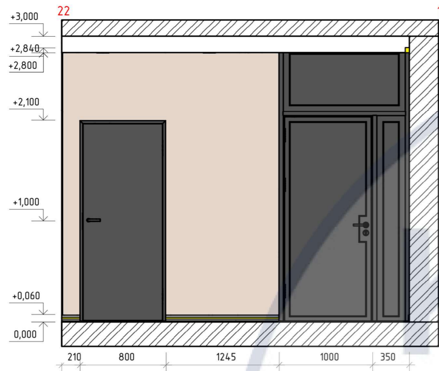
Розгортка 22-1 M1:40
