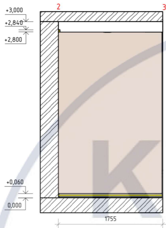
Розгортка 2-3 M1:40
