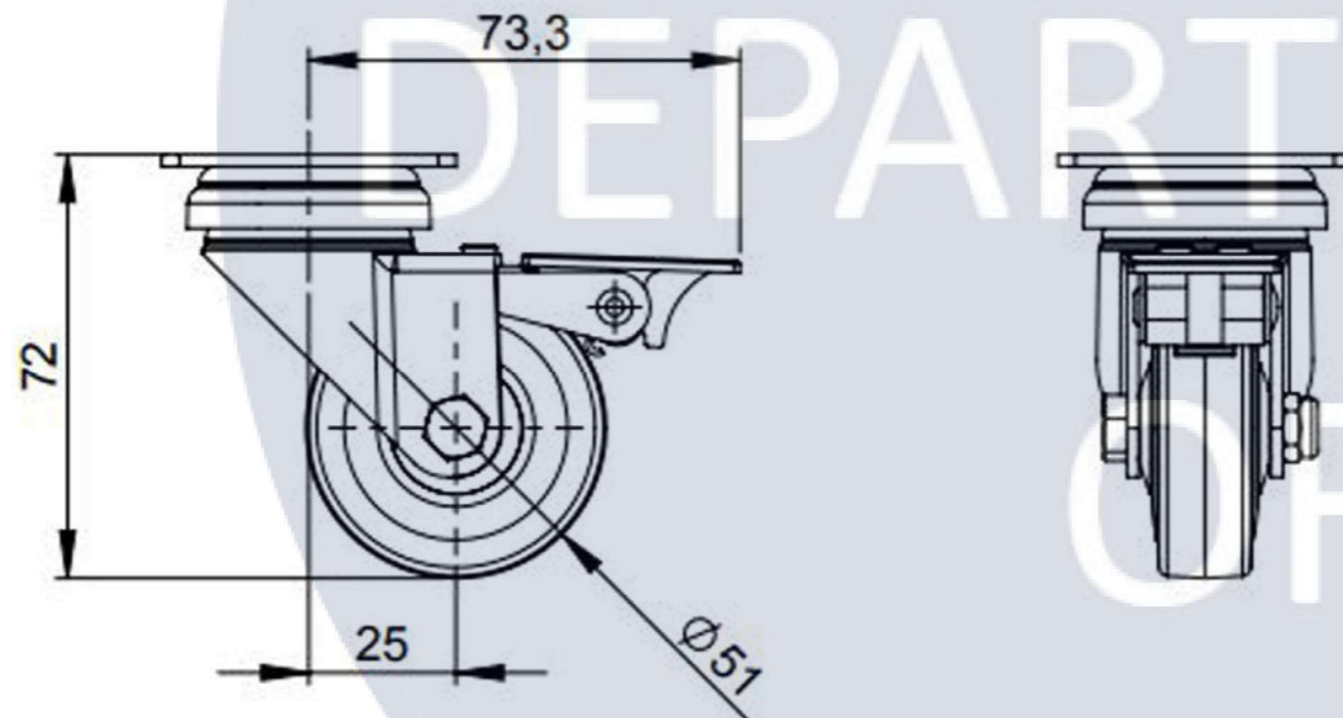
Коліщатка меблева поворотна з фіксатором
