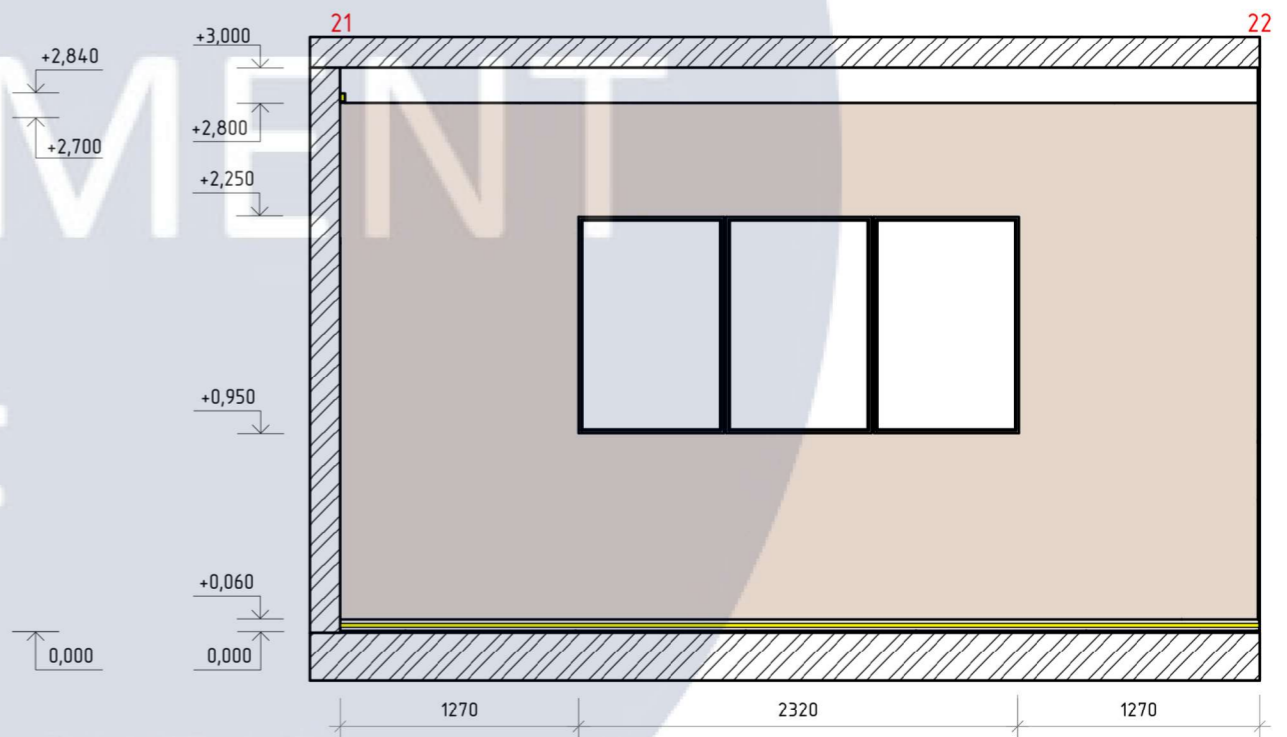
Розгортка 21-22 M1:40
