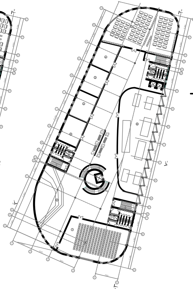
ПЛАН ТРЕТЬОГО ПОВЕРХУ
