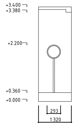
Розгортка 12-1
