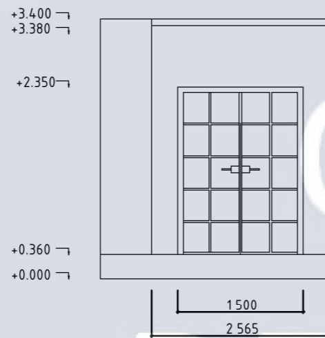
Розгортка 8-9
