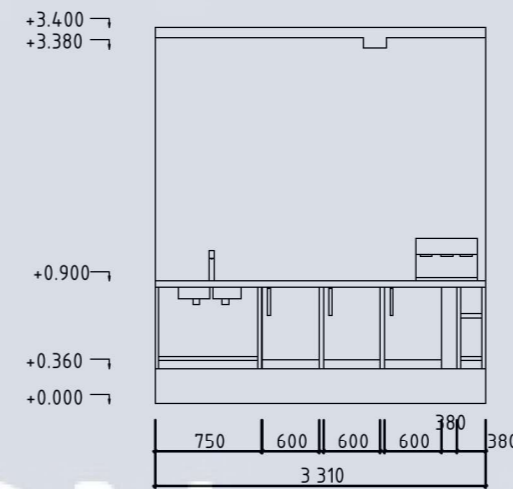
Розгортка 10-11
