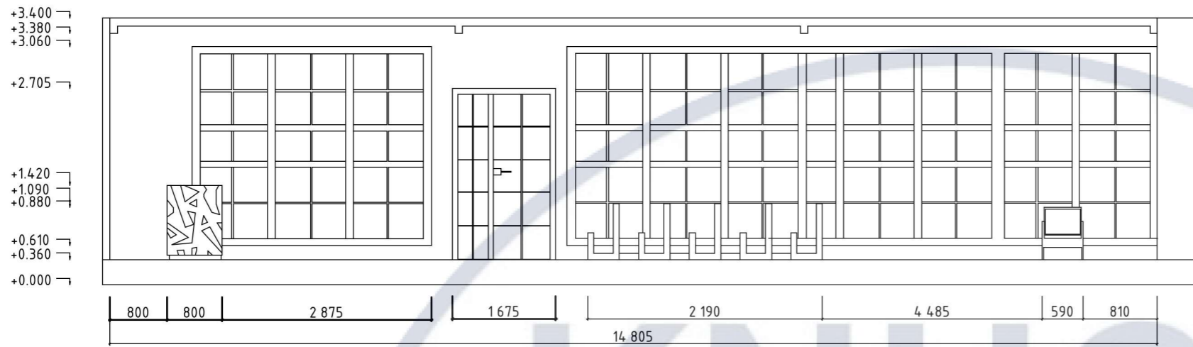
Розгортка 1-2
