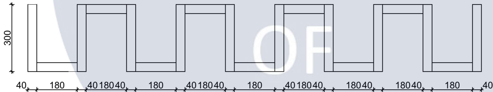
Вид зверху
