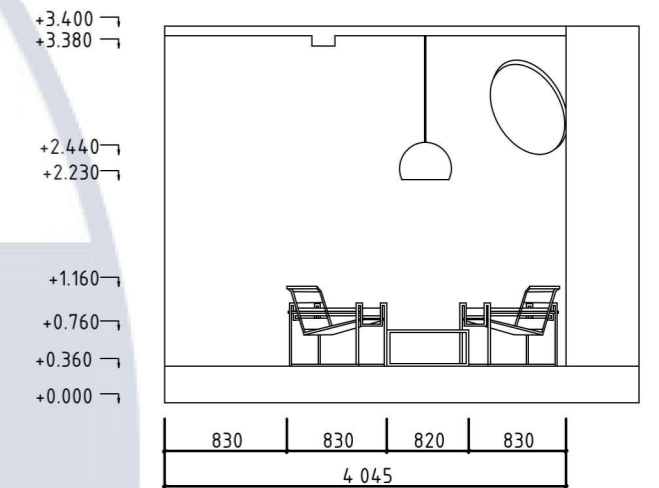
Розгортка 6-7
