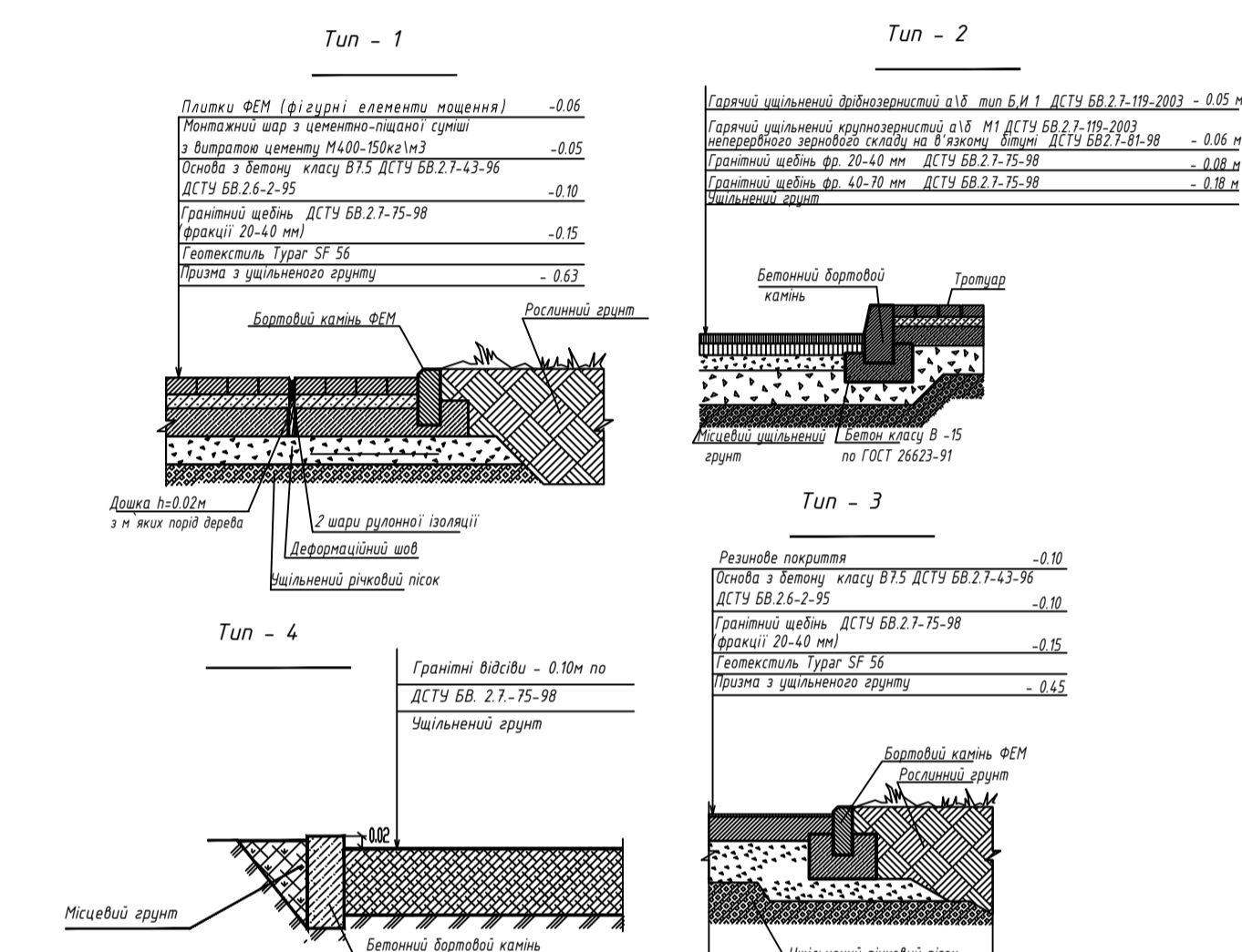
Конструкції покриття
