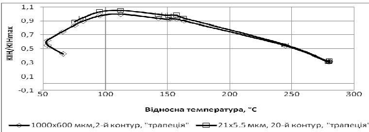
Рис. 6. Температурна залежність відносних значень КІІ в найбільш глибокій точці тріщини: a – в задачі теорії пружності; b – в задачі теорії пластичності без урахування історії навантаження
