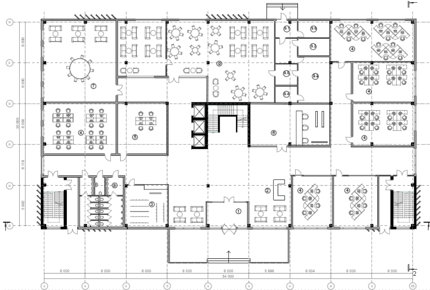
ПЛАН ПЕРШОГО ПОВЕРХУ
