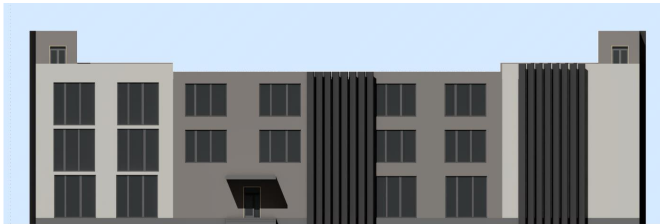
ФАСАД В ОСЯХ 10-1
