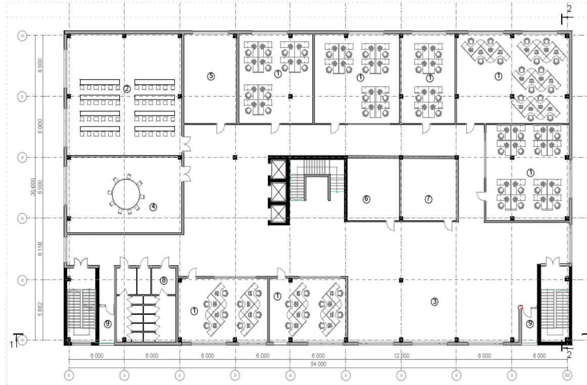
ПЛАН ТРЕТЬОГО ПОВЕРХУ
