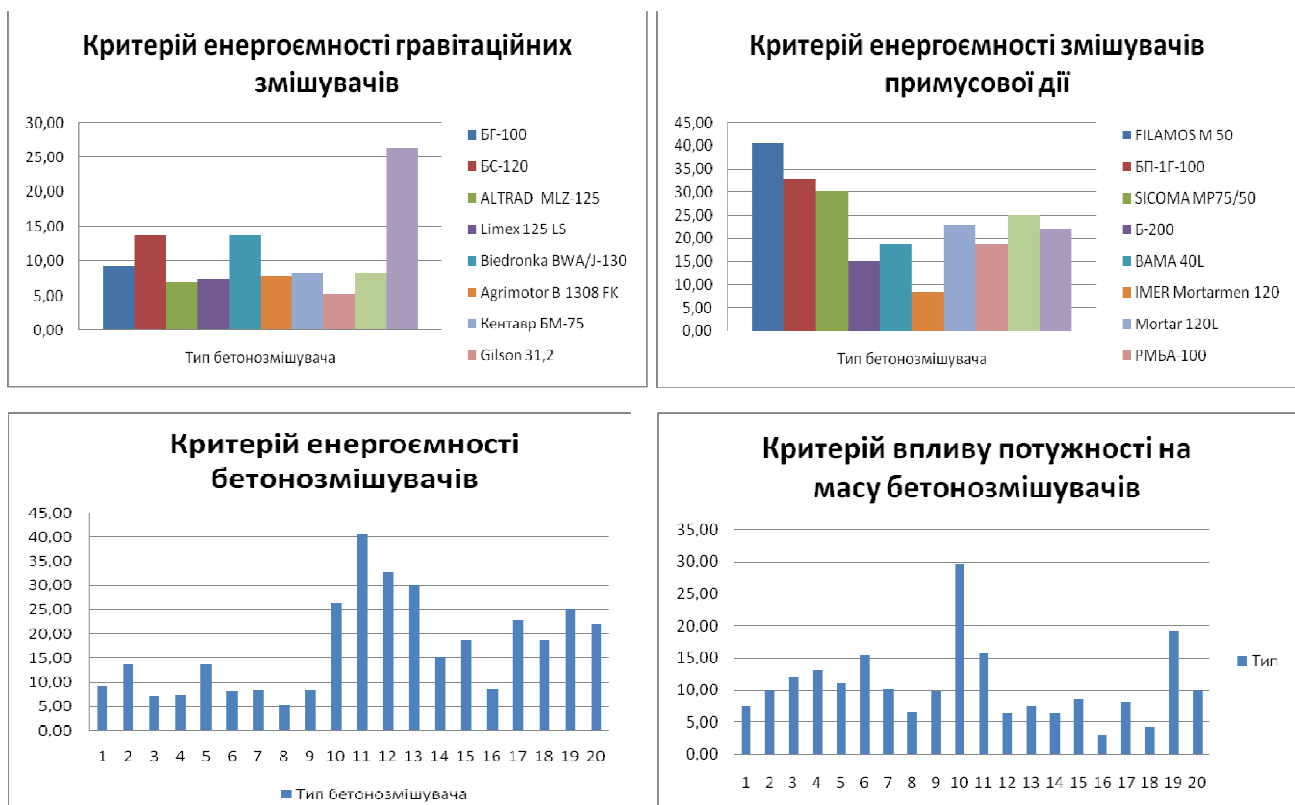
Рис. 3. Гістограми зміни критеріїв енергоємності бетонозмішувачів різних типів.
