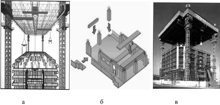
Рис. 2. Загальний вигляд проекту Big-Canopy (а), його просторова модель (б) та фото реального будівництва (в).
