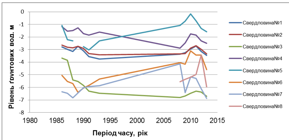
Рис.3. Зведений графік рівнів ґрунтових вод Херсонського регіону по свердловинах № 1-8
