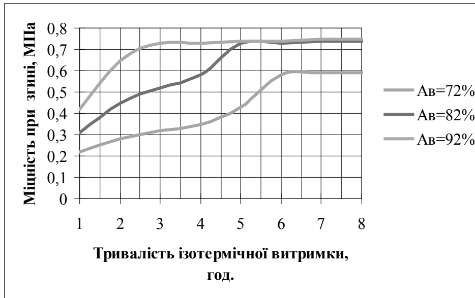
Рисунок 5 - Динаміка росту міцності при згині автоклавного газобетону в залежності від активності використаного вапна
