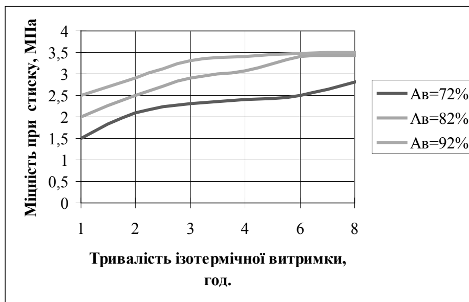
Рисунок 4 - Динаміка росту міцності при стиску автоклавного газобетону в залежності від активності використаного вапна
