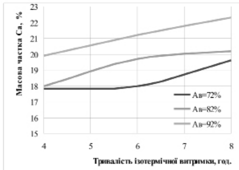
Рисунок 1 - Кінетика зв'язування СаО за автоклавної обробки в залежності від активності використаного вапна
