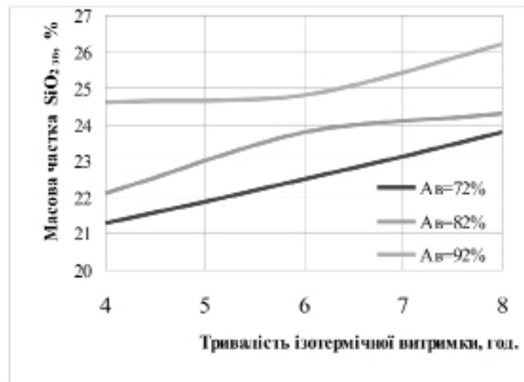
Рисунок 2 - Кінетика зв'язування SiO 2 за автоклавної обробки в залежності від активності використаного вапна
