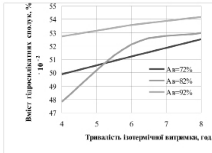
Рисунок 3 - Кінетика синтезу гідросилікатів кальцію в складі автоклавного газобетону залежно від активності використаного вапна
