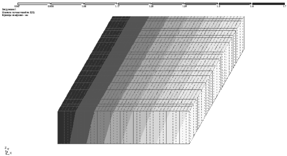
Рис.8. Изополя перемещень уздовж осі Z, мм перерізу 2-2 залізобетонної колони при прогріві для пожежі тривалістю 90 хв.
