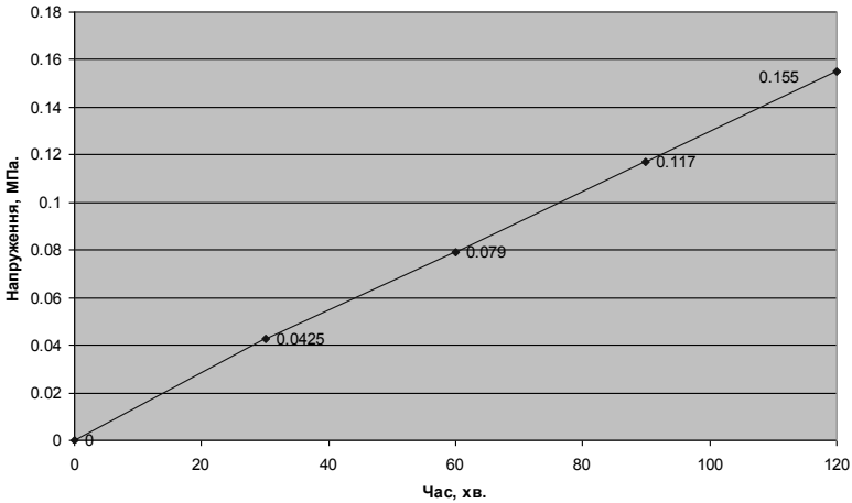
Рис. 14. Графік залежності напружень \tau_{xy} , МПа елеента №780 в залежності від впливу температури стандартної пожежі.
