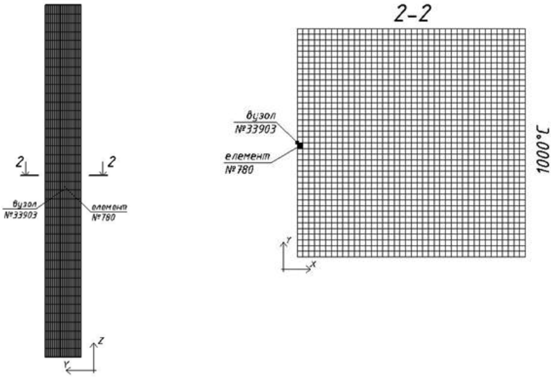
Рис. 4. Схема розміщення вузлів та скінченних елементів колони.
