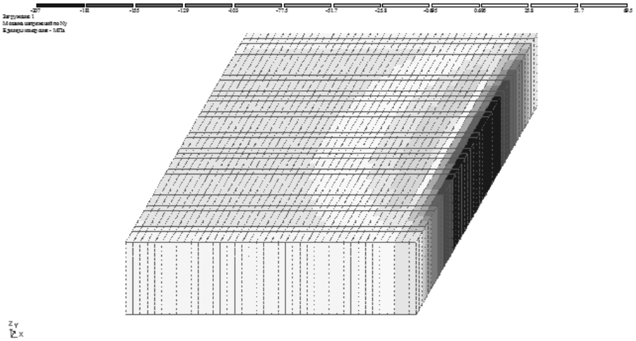
Рис.9. Ізополя напружень \sigma_y , МПа перерізу 2-2 залізобетонної колони при прогріві для пожежі тривалістю 90 хв.
