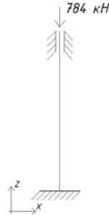
Рис. 2. Розрахункова схема защемлення колони.
