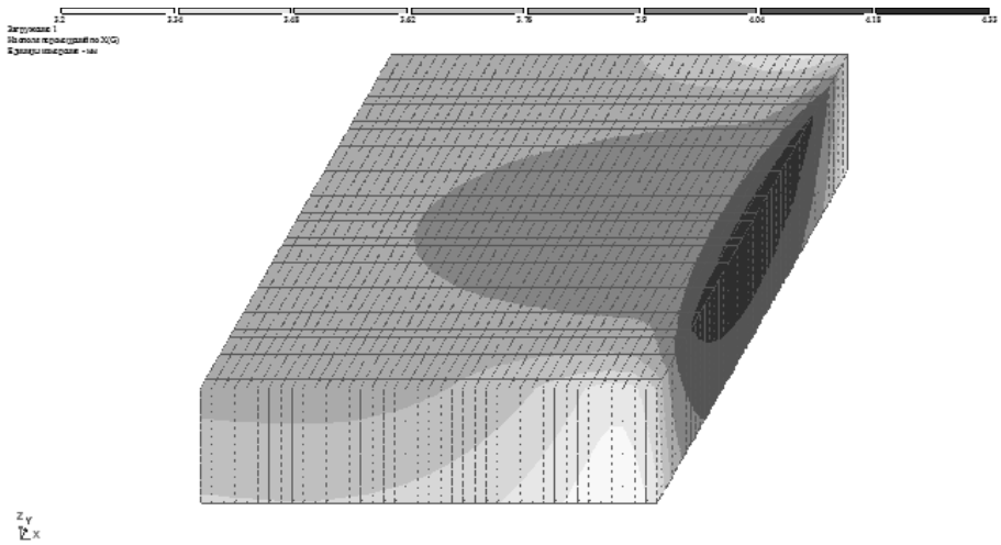
Рис.7. Изополя перемещень уздовж осі X, мм перерізу 2-2 залізобетонної колони при прогріві для пожежі тривалістю 90 хв.
