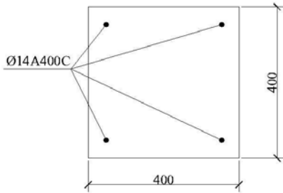
Рис. 1. Розрахунковий переріз колони.
