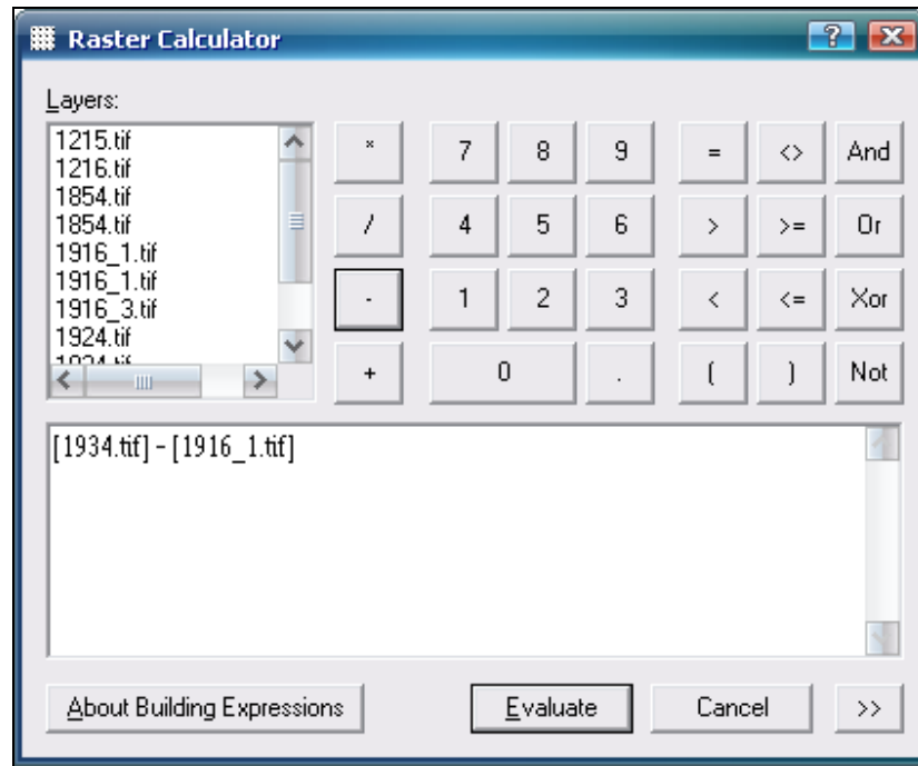
Рис. 3.2.11. Калькулятор растрів
