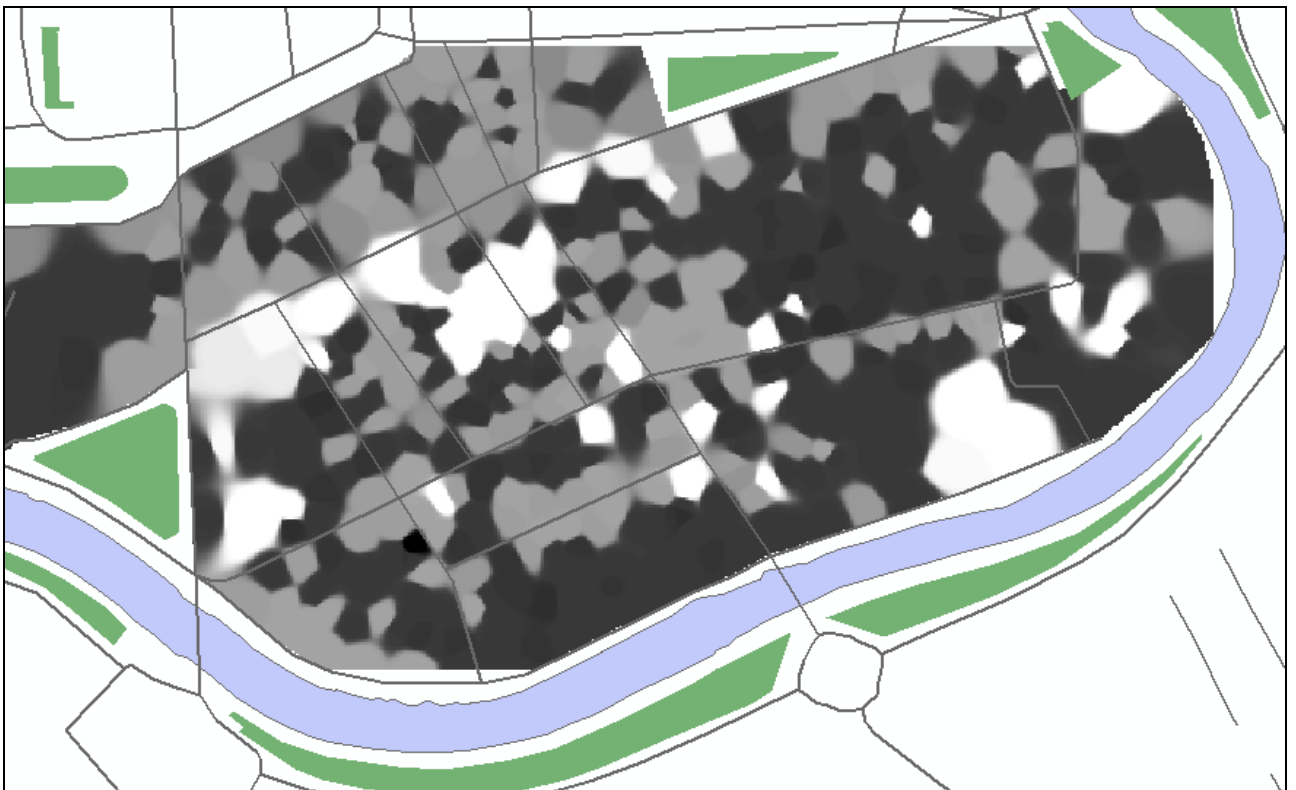
Рис. 3.2.12 Результуочий ґрід
