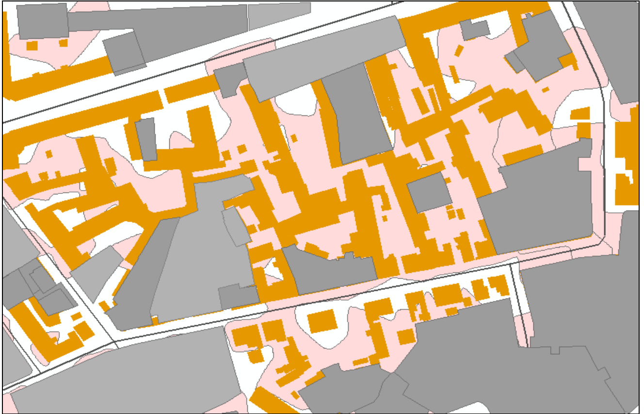
Рис. 3.2.20 Кінцевий ґрид
