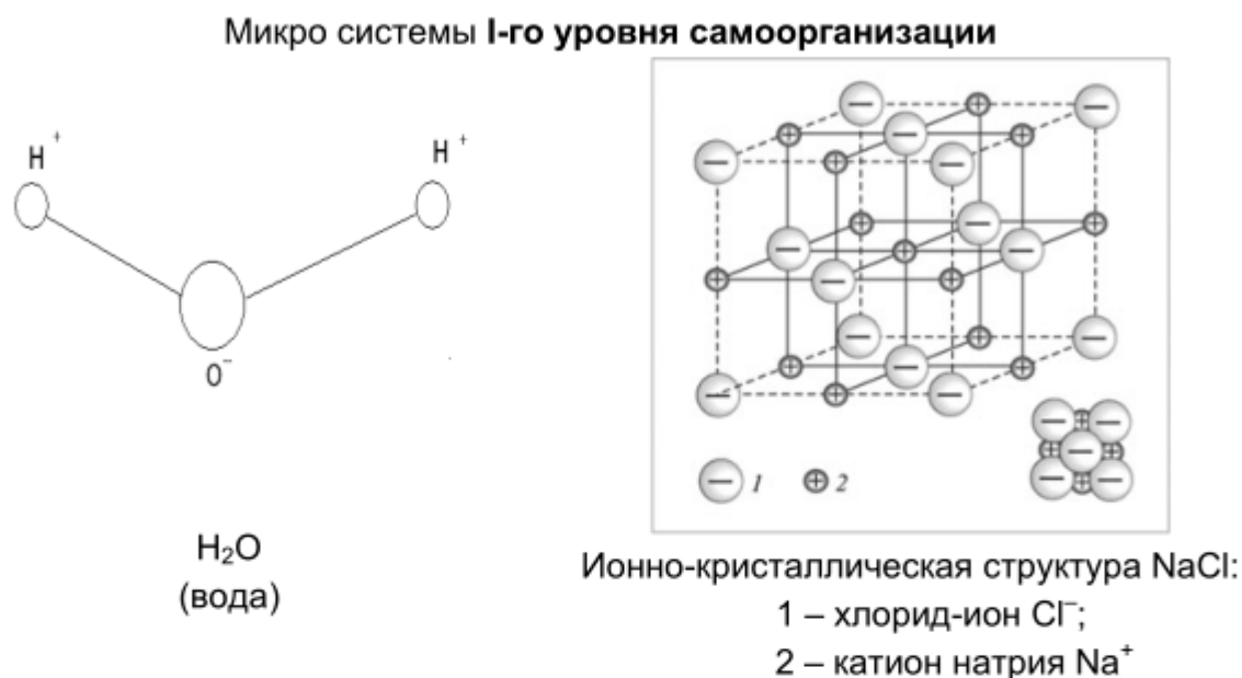
Рис.3. Примеры самоорганизованных микросистем I-го уровня.
