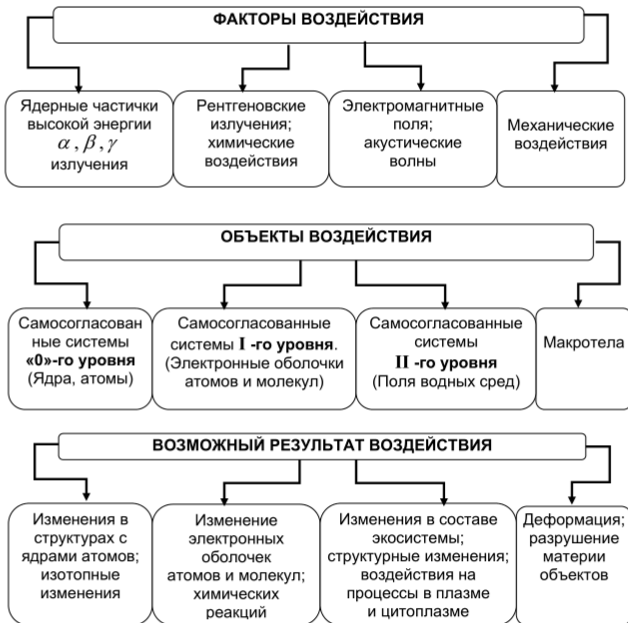
Рис.7. Техногенные воздействия и структурные особенности материи.
