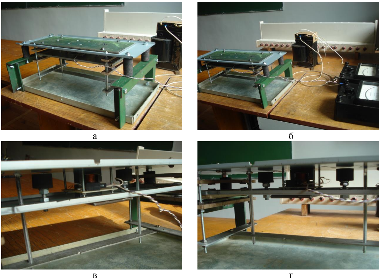
Рисунок 7. Лабораторна двомасова електромагнітна ударно-вібраційна установка зі зміненою конструкцією підвіски ударника.
