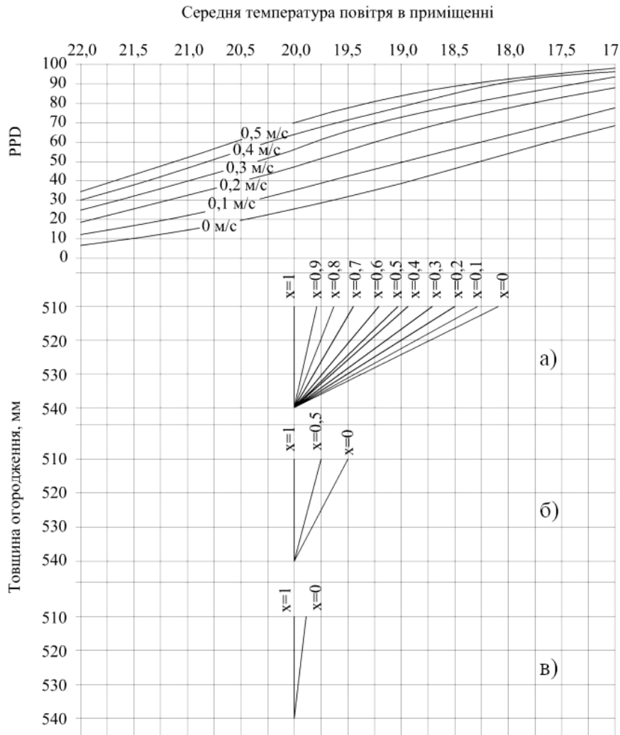
Рис. 2. Прогнозований відсоток незадоволених температурним середовищем (PPD) в залежності від ступеня дефекту зовнішньої огорожуючої конструкції: а) за умови наявності дефектної зони тільки зовнішньої стіни [8]; б) за умови наявності дефектної зони зовнішньої стіни з вбудованим в нього вікном [11]; в) за умови наявності декількох різнотипових огорожуючих конструкцій та дефектної зони зовнішньої стіни з вбудованим в нього вікном [11]
