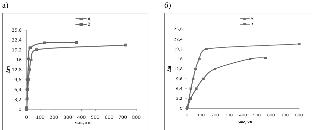
Рисунок 3. Кінетика капілярного просочування штучного каменю: а) ГЦПВ; б) модифікованої ГЦПВ
