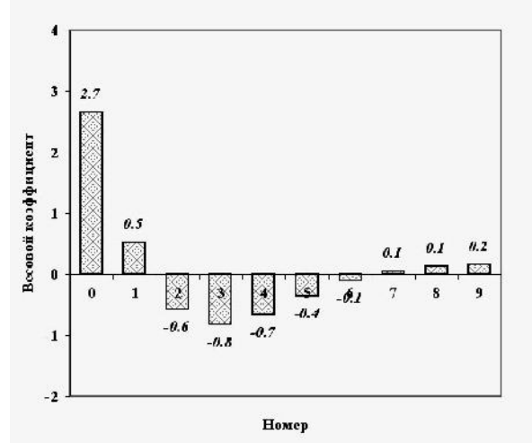
Рис. 2. Весовая функция динамического корректора (массив весовых коэффициентов)
