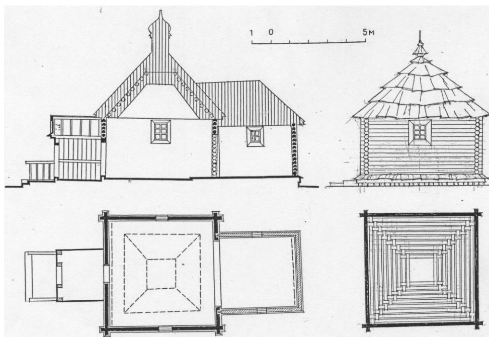
Рис.2. Каплиця у с.Дроздині на Рівненщині: ліворуч – план і розріз після перебудови кін. XIX – поч. XX ст.; праворуч – південний фасад та план перекриття до перебудови (реконструкція В.Завади).
