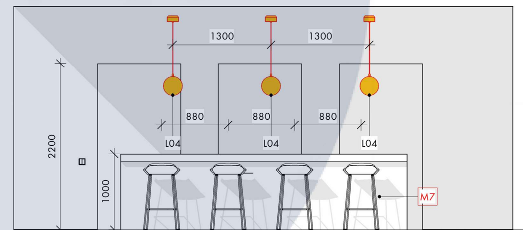
2-3 ресепшн 1 : 50
