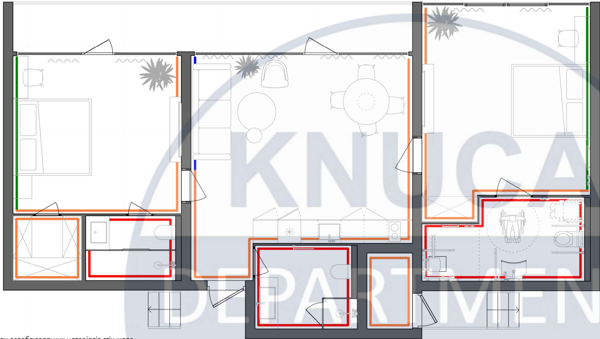
План оздоблювальних матеріалів стін шале 1 : 60
