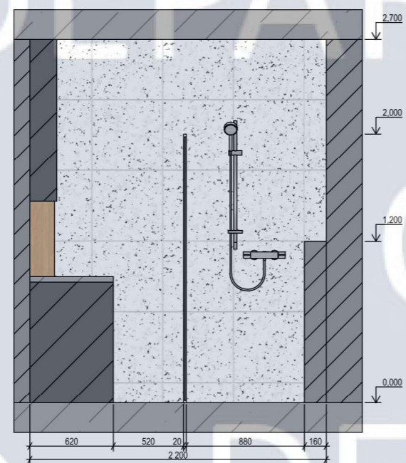
Розгортка 10-11 М 1:40
