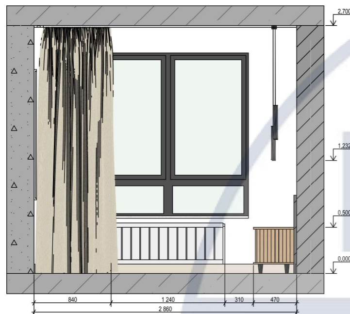
Розгортка 5-6 М 1:40
