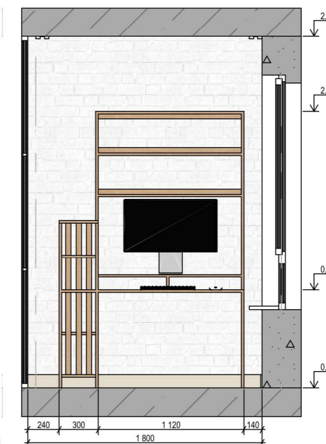
Розгортка 4-1 М 1:40
