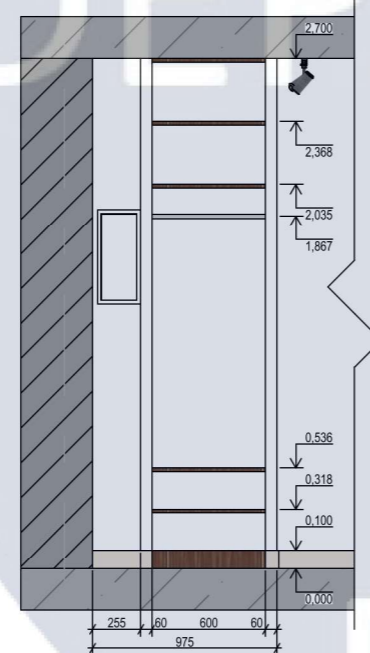
Розгортка 18-19 М 1:40
