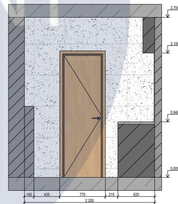
Розгортка 12-9 М 1:40
