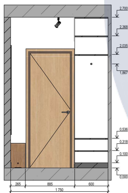
Розгортка 17-20 М 1:40
