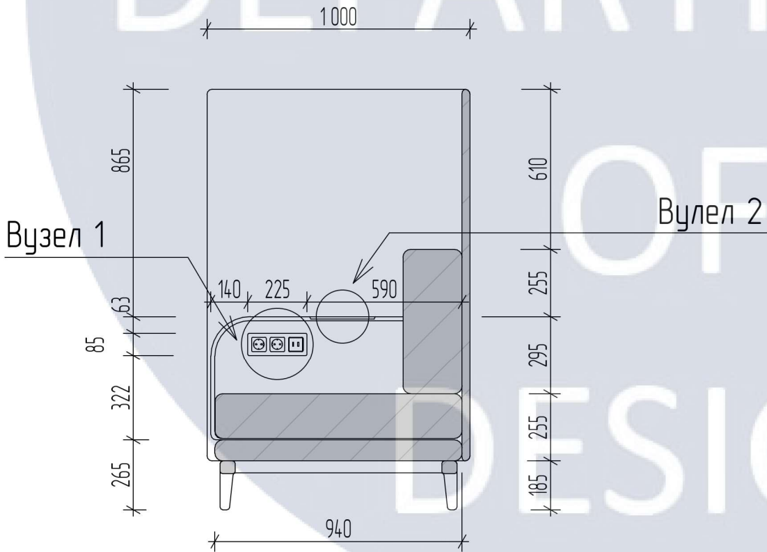
Розріз А-А. М 1:20
