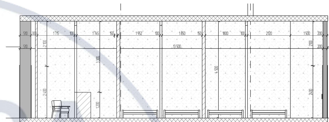
Читальна зала. Рохріз Б-Б
