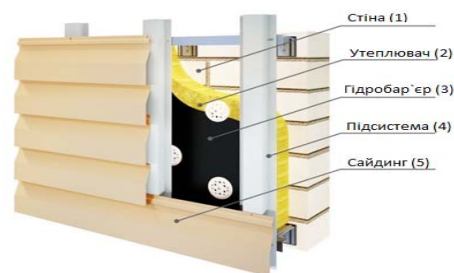
Рисунок 1. Облицювання полівінілхлоридними сайдинговими панелями
